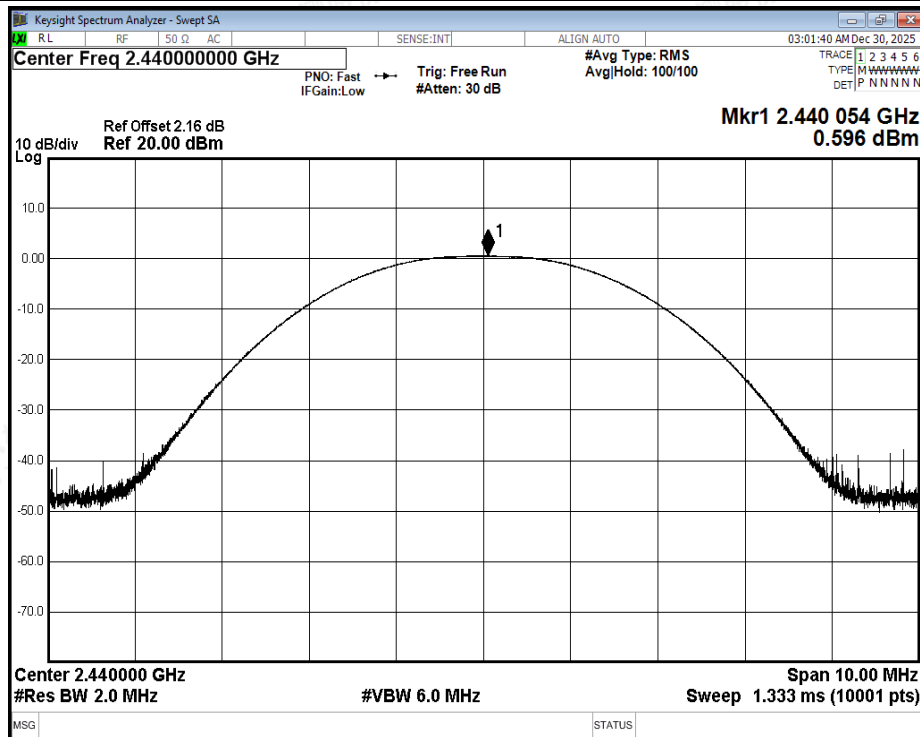
Power NVNT BLE 2440MHz Ant
