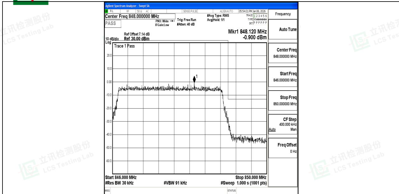
Band5_3MHz_16QAM_20635_15RB#0
