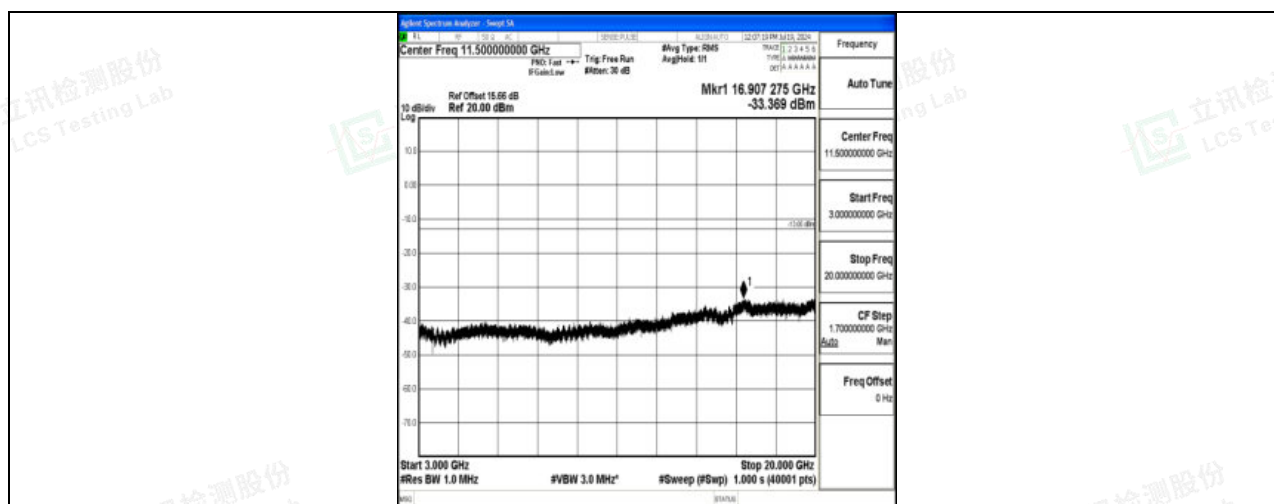
Band2 10MHz 16QAM 19150 1RB#0 3000~20000 3000~20000
