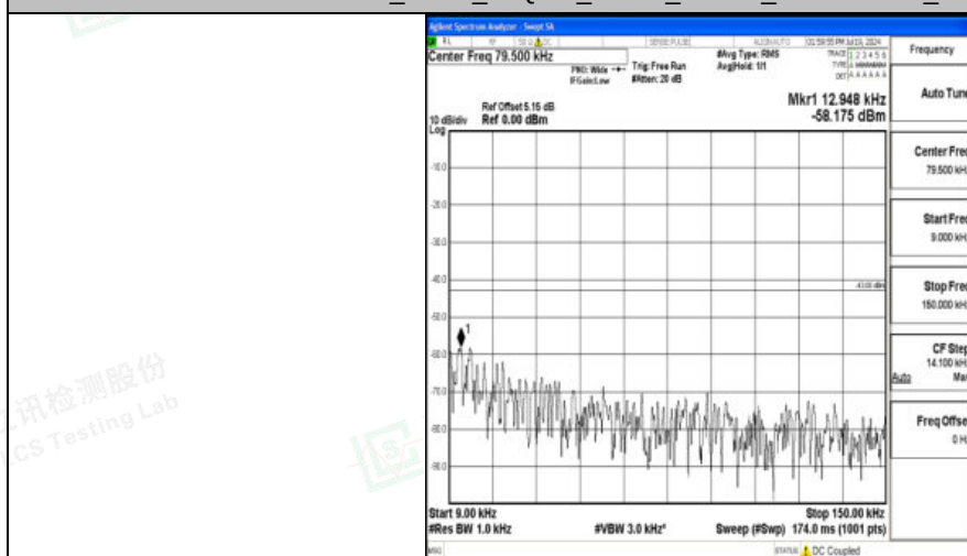
Band4 5MHz QPSK 20375 1RB#0 0.009~0.15 0.009~0.15
