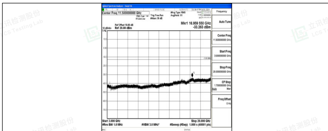
Band4 3MHz 16QAM 20175 1RB#0 3000~20000 3000~20000
