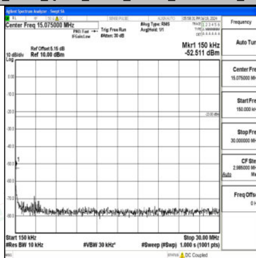
Band12 5MHz QPSK 23035 1RB#0 0.15~30 0.15~30
