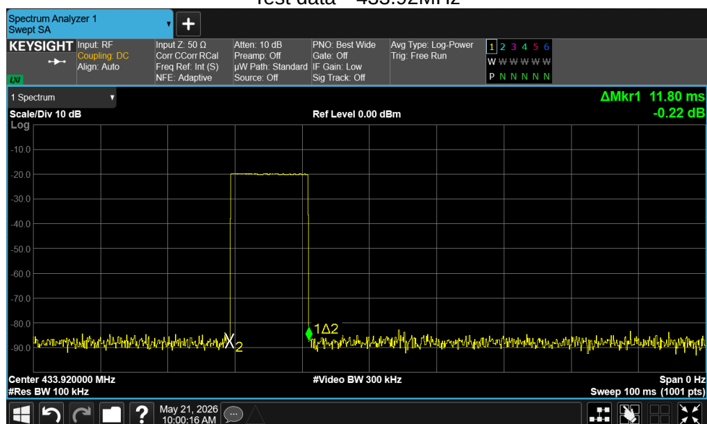
Test data—433.92MHz
