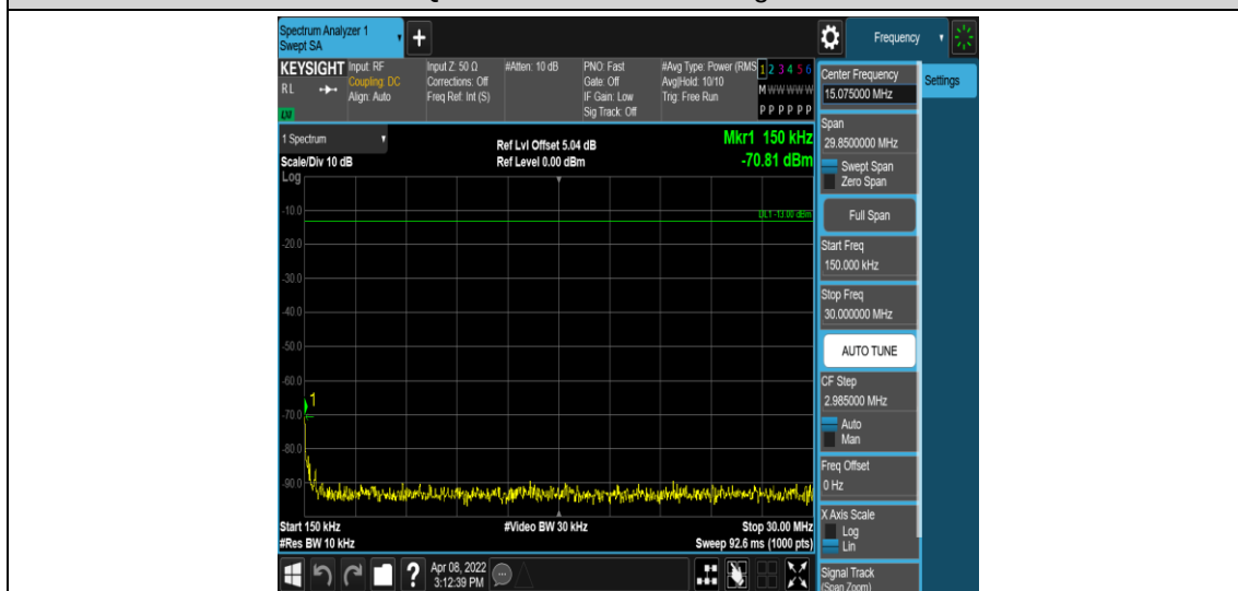
Band2-5MHz-QPSK-18900-1RB#0-Range2:0.15~30MHz
