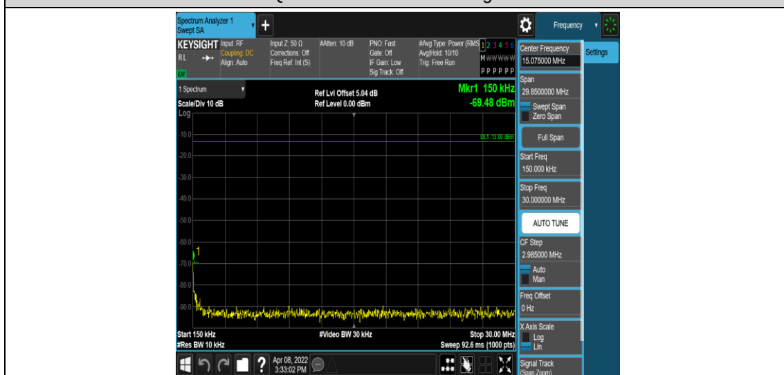
Band2-10MHz-QPSK-18900-1RB#0-Range2:0.15~30MHz
