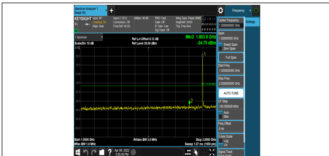
Band2-10MHz-QPSK-19150-1RB#0-Range4:1000~2000MHz
