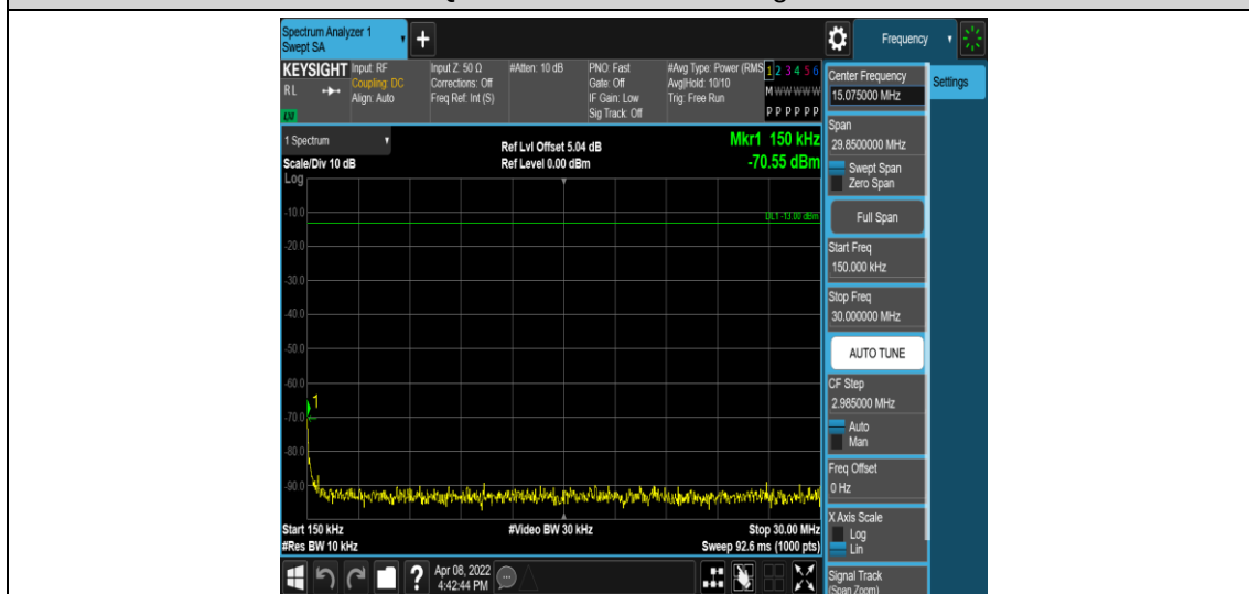
Band4-1.4MHz-QPSK-20393-1RB#0-Range2:0.15~30MHz
