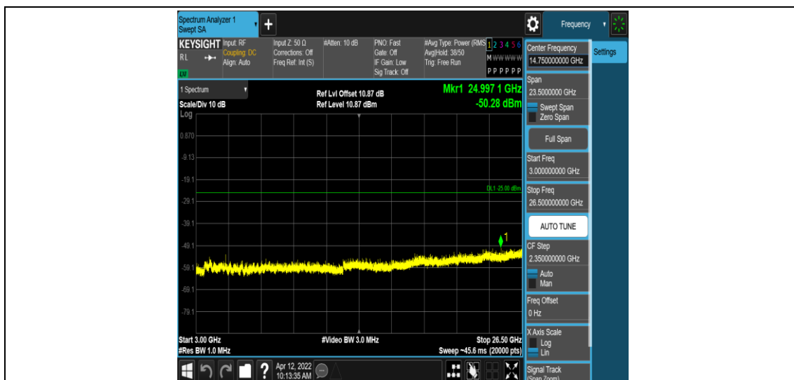
Band7-5MHz-QPSK-21425-1RB#0-Range5:3000~26500MHz
