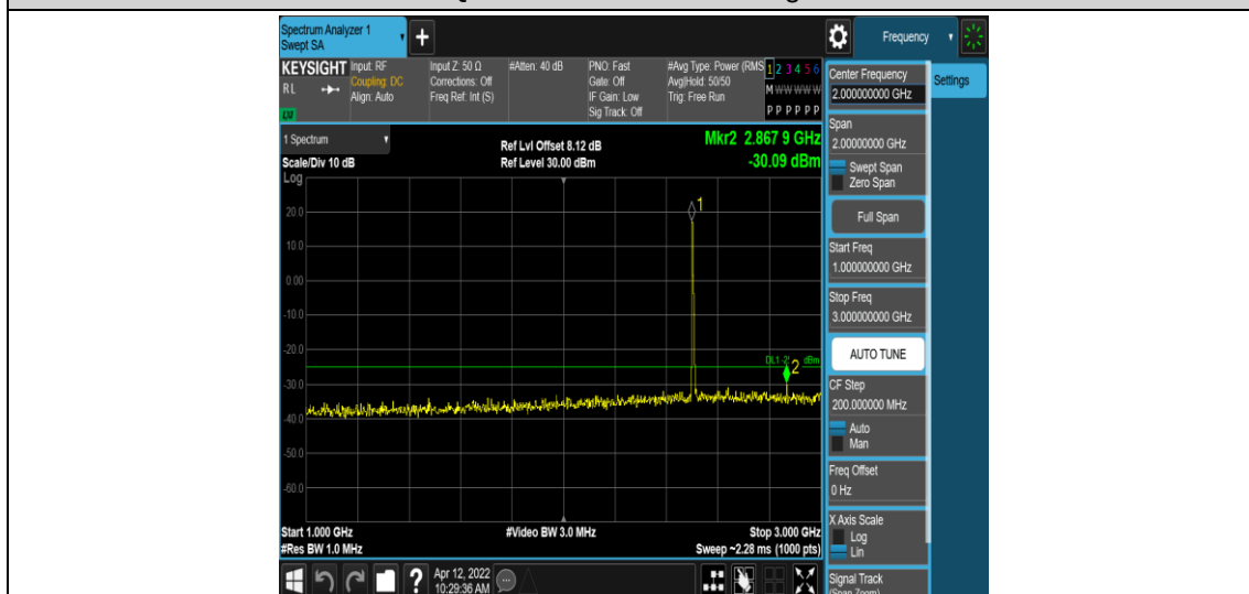
Band7-10MHz-QPSK-20800-1RB#0-Range4:1000~3000MHz
