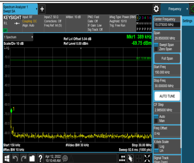
Band7-5MHz-QPSK-21100-1RB#0-Range2:0.15~30MHz
