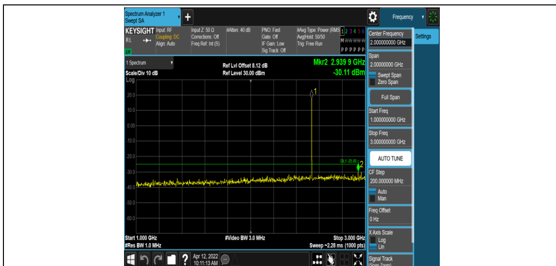
Band7-5MHz-QPSK-21100-1RB#0-Range4:1000~3000MHz
