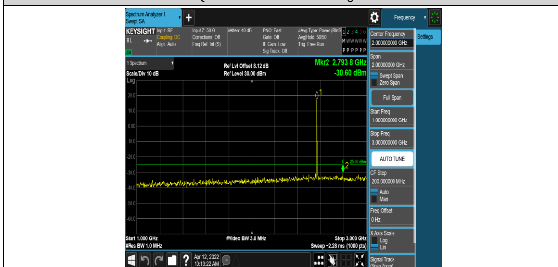
Band7-5MHz-QPSK-21425-1RB#0-Range4:1000~3000MHz
