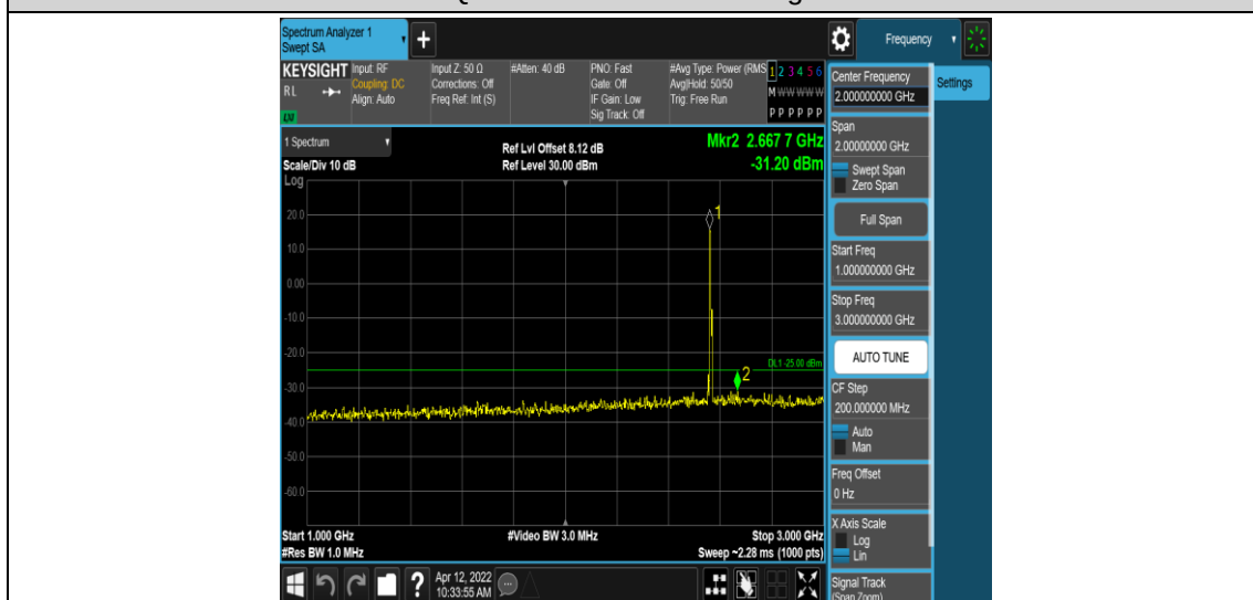
Band7-10MHz-QPSK-21400-1RB#0-Range4:1000~3000MHz
