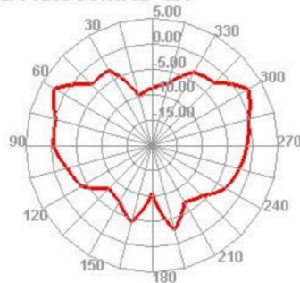
2442.000MHz E1
