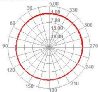
2442.000MHz H
