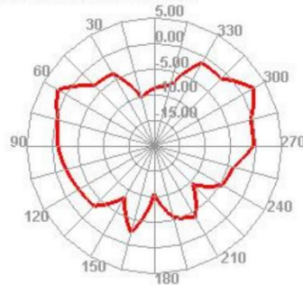
2442.000MHz E2
