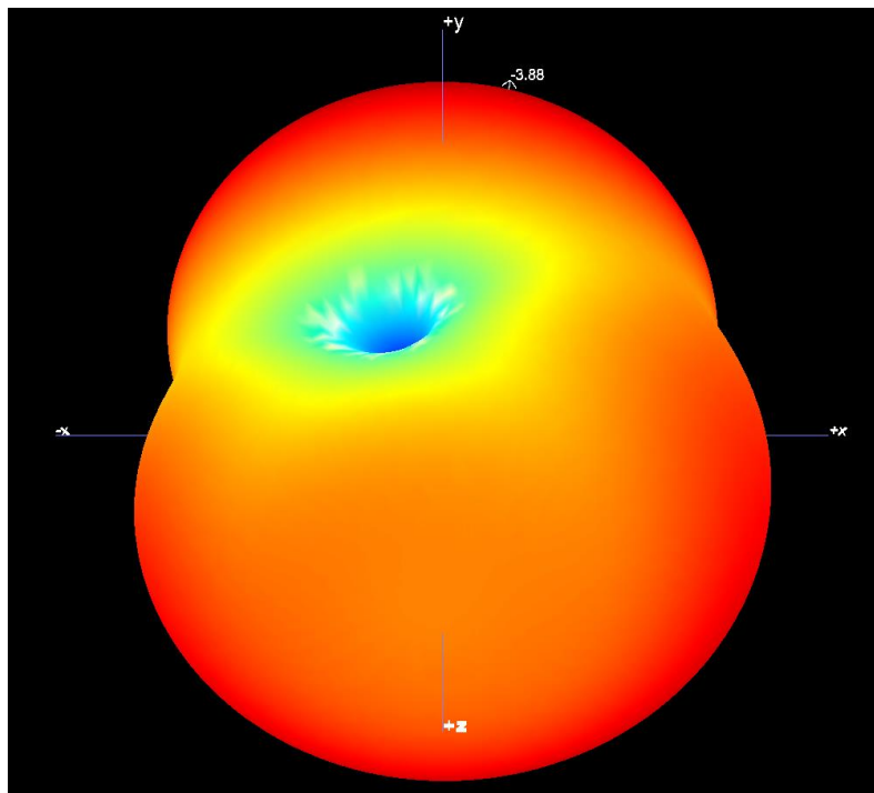
B1.4 3D Pattern for 440MHz
