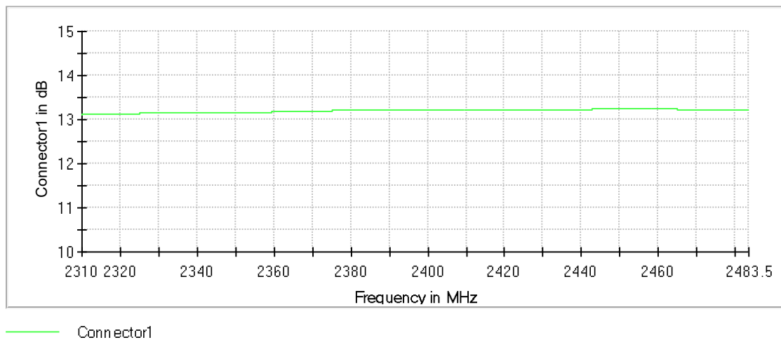
Attenuation
