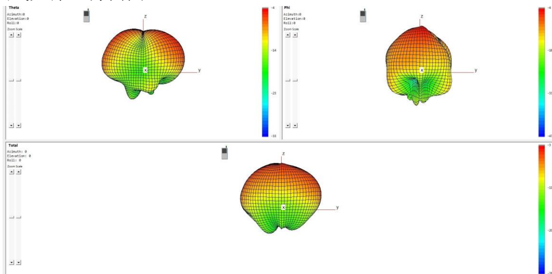
天线无源3D方向图（BT5.0）
