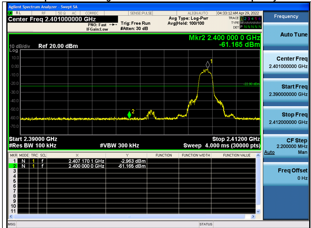
Test_Graph_GFSK_ANT1_2407_Lower Band Edge Emissions
