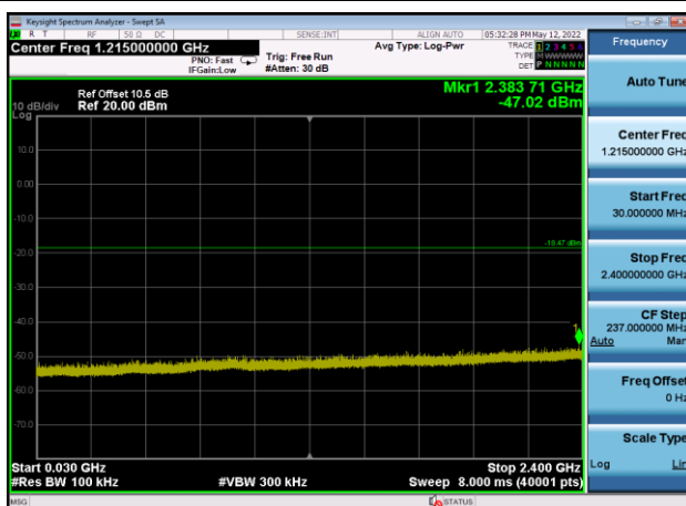
,Plot 3,30MHz~2400MHz-802.11n(HT20) ,2462MHz,Ant9
