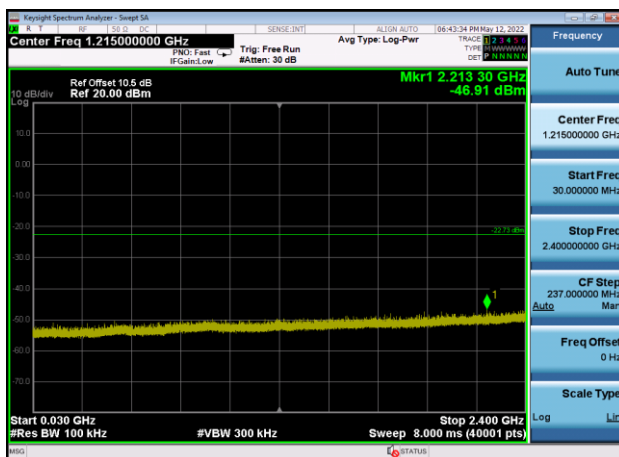
,Plot 3,30MHz~2400MHz-802.11n(HT40) ,2452MHz,Ant9
