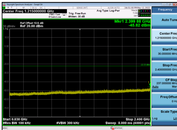
,Plot 3,30MHz~2400MHz-802.11n(HT40) ,2437MHz,Ant9
