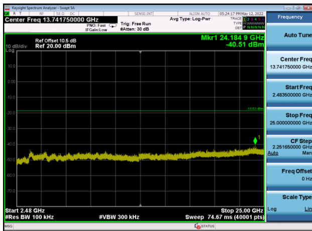
,Plot 4,2483.5MHz~25000MHz-802.11n(HT 20),2462MHz,Ant9
