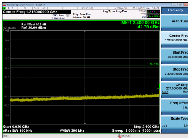
,Plot 3,30MHz~2400MHz-802.11n(HT20) ,2437MHz,Ant9
