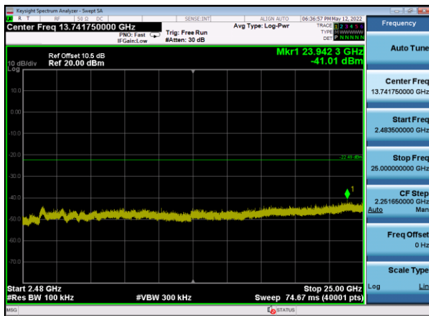
,Plot 4,2483.5MHz~25000MHz-802.11n(HT 40),2452MHz,Ant9
