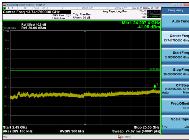
,Plot 4,2483.5MHz~25000MHz-802.11n(HT 40),2437MHz,Ant9
