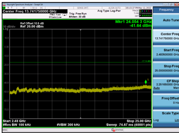
,Plot 4,2483.5MHz~25000MHz-802.11n(HT 20),2437MHz,Ant9
