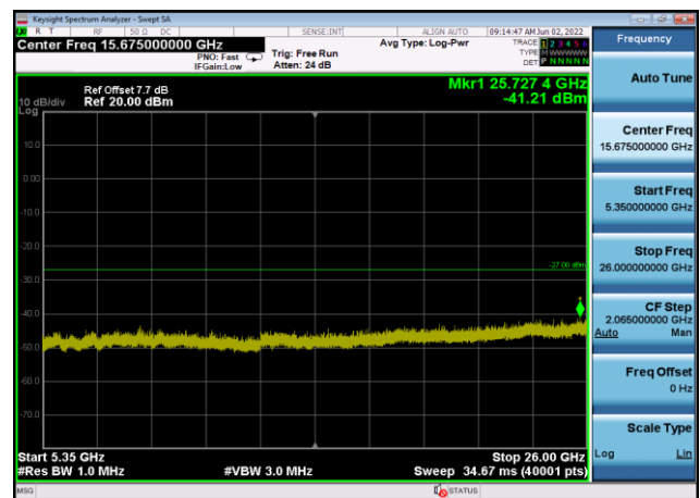
U-NII-1 ,Plot 3,5350MHz~26000MHz-802. 11n(20MHz),5240MHz,Ant8
