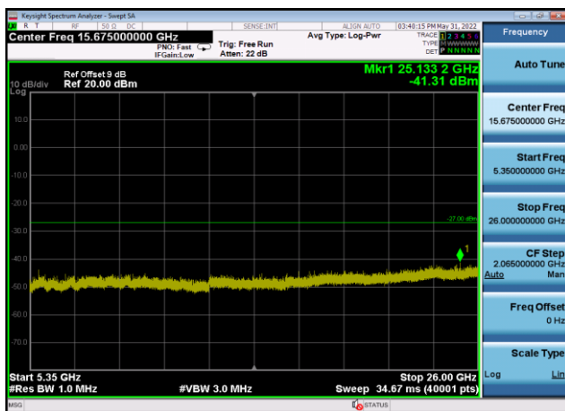
U-NII-1 ,Plot 3,5350MHz~26000MHz-802. 11ac(20MHz),5240MHz,Ant9
