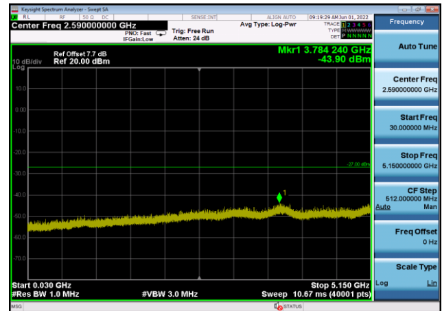
U-NII-1 ,Plot 2,30MHz~5150MHz-802.11a (20MHz),5220MHz,Ant8
