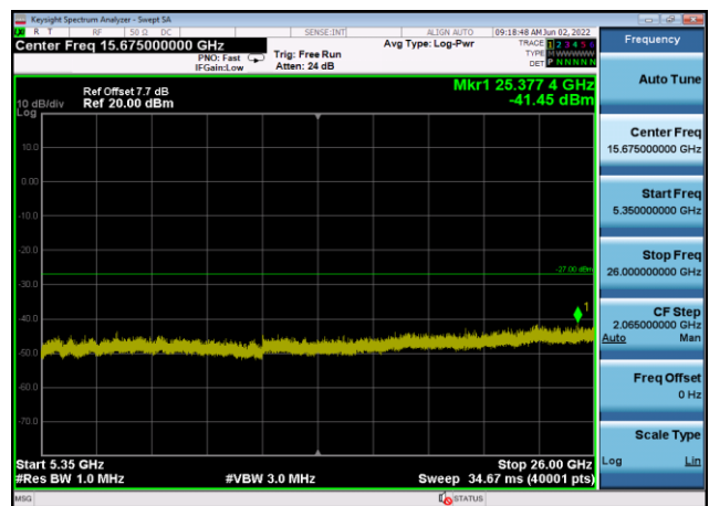
U-NII-1 ,Plot 3,5350MHz~26000MHz-802. 11ac(20MHz),5240MHz,Ant8
