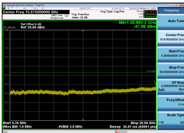
U-NII-1 ,Plot 3,5350MHz~26000MHz-802. 11ax(20MHz),5240MHz,Ant9
