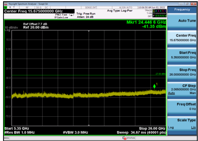
U-NII-1 ,Plot 3,5350MHz~26000MHz-802. 11ac(80MHz),5210MHz,Ant8
