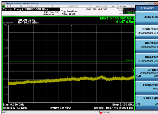
U-NII-1 ,Plot 2,30MHz~5150MHz-802.11a (20MHz),5220MHz,Ant9
