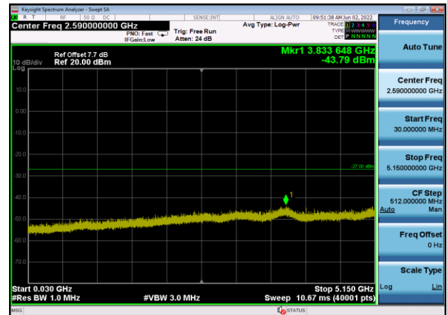
U-NII-1 ,Plot 2,30MHz~5150MHz-802.11a x(40MHz),5230MHz,Ant8
