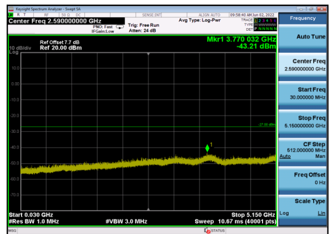
U-NII-1 ,Plot 2,30MHz~5150MHz-802.11a c(80MHz),5210MHz,Ant8
