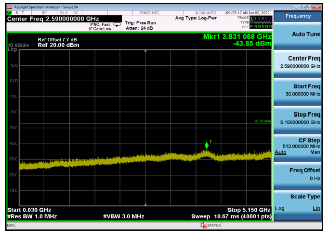
U-NII-1 ,Plot 2,30MHz~5150MHz-802.11a c(20MHz),5220MHz,Ant8
