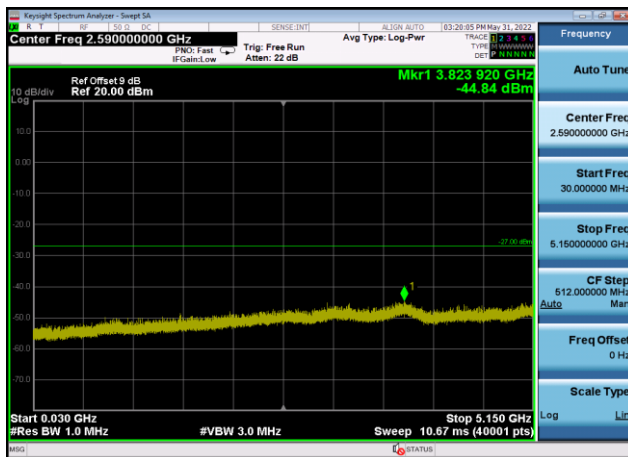
U-NII-1 ,Plot 2,30MHz~5150MHz-802.11a (20MHz),5240MHz,Ant9
