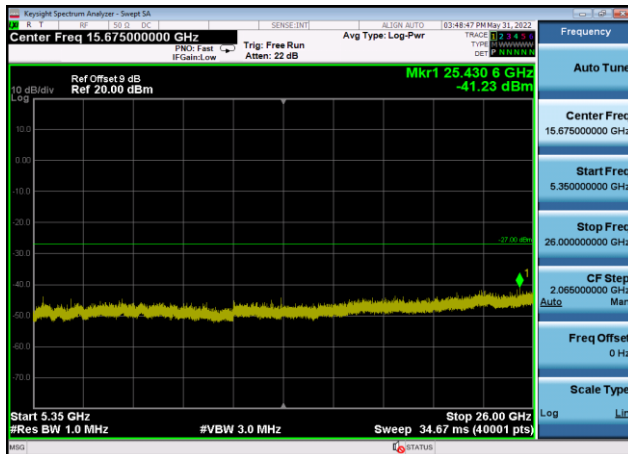
U-NII-1 ,Plot 3,5350MHz~26000MHz-802. 11ax(20MHz),5220MHz,Ant9
