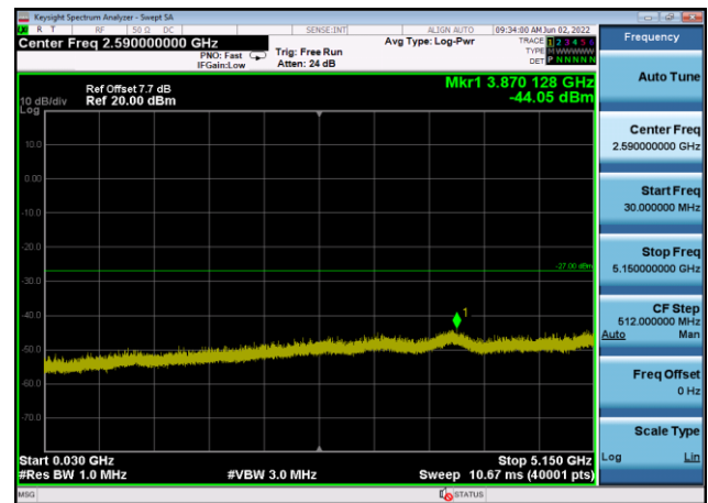
U-NII-1 ,Plot 2,30MHz~5150MHz-802.11a x(20MHz),5240MHz,Ant8
