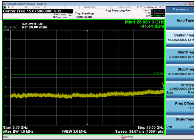
U-NII-1 ,Plot 3,5350MHz~26000MHz-802. 11ac(80MHz),5210MHz,Ant9
