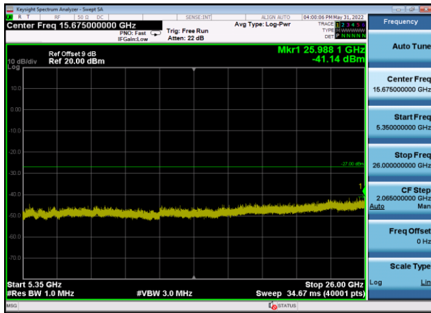
U-NII-1 ,Plot 3,5350MHz~26000MHz-802. 11ac(40MHz),5230MHz,Ant9
