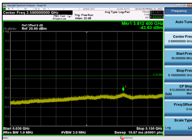
U-NII-1 ,Plot 2,30MHz~5150MHz-802.11a x(20MHz),5240MHz,Ant9
