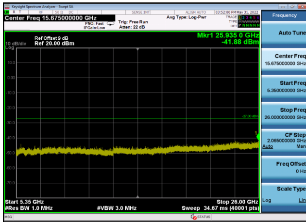
U-NII-1 ,Plot 3,5350MHz~26000MHz-802. 11ax(40MHz),5230MHz,Ant9
