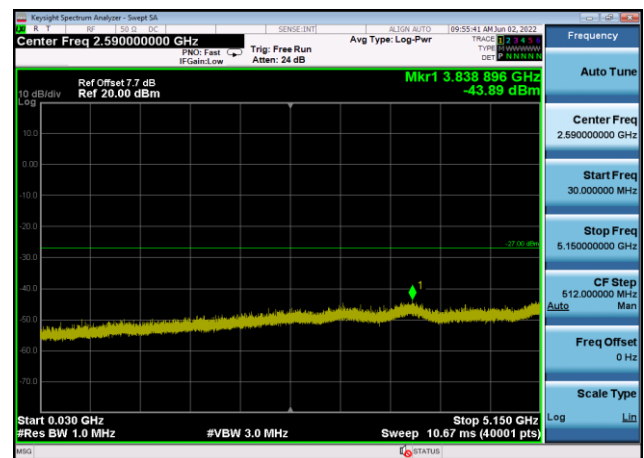
U-NII-1 ,Plot 2,30MHz~5150MHz-802.11a x(80MHz),5210MHz,Ant8
