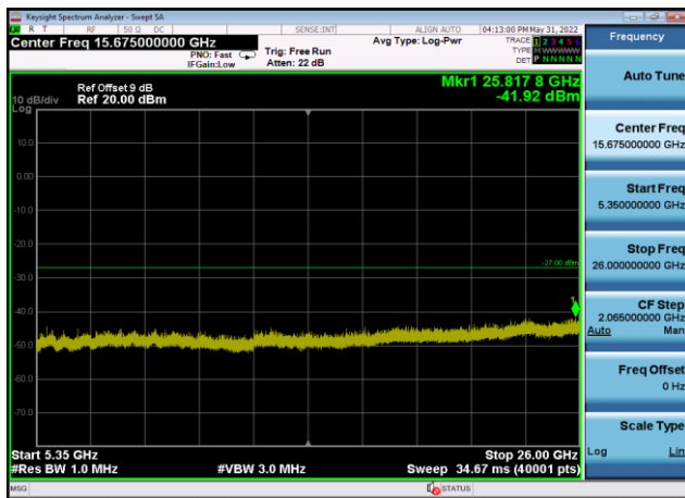
U-NII-1 ,Plot 3,5350MHz~26000MHz-802. 11ax(80MHz),5210MHz,Ant9
