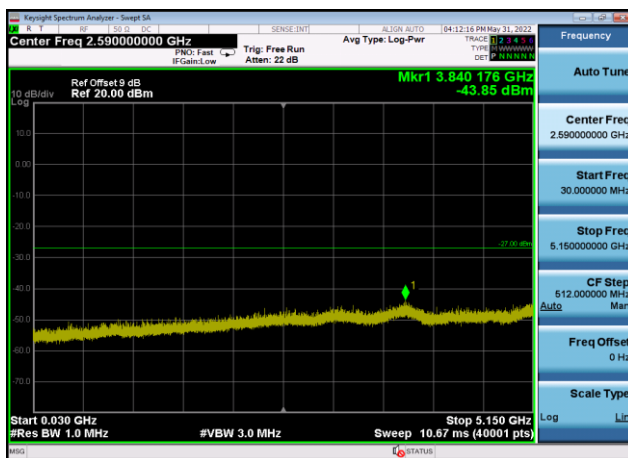
U-NII-1 ,Plot 2,30MHz~5150MHz-802.11a x(80MHz),5210MHz,Ant9
