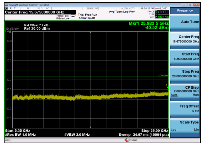
U-NII-1 ,Plot 3,5350MHz~26000MHz-802. 11ax(80MHz),5210MHz,Ant8
