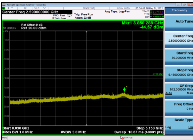
U-NII-1 ,Plot 2,30MHz~5150MHz-802.11a c(20MHz),5240MHz,Ant9
