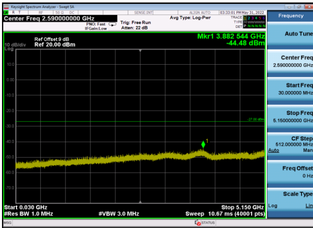
U-NII-1 ,Plot 2,30MHz~5150MHz-802.11a c(20MHz),5220MHz,Ant9
