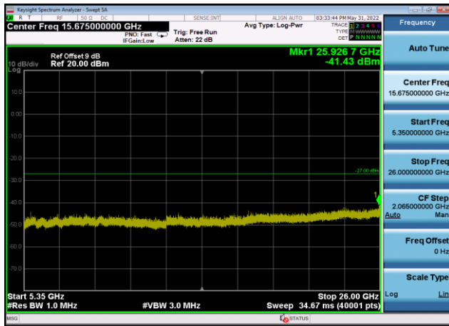
U-NII-1 ,Plot 3,5350MHz~26000MHz-802. 11ac(20MHz),5220MHz,Ant9
