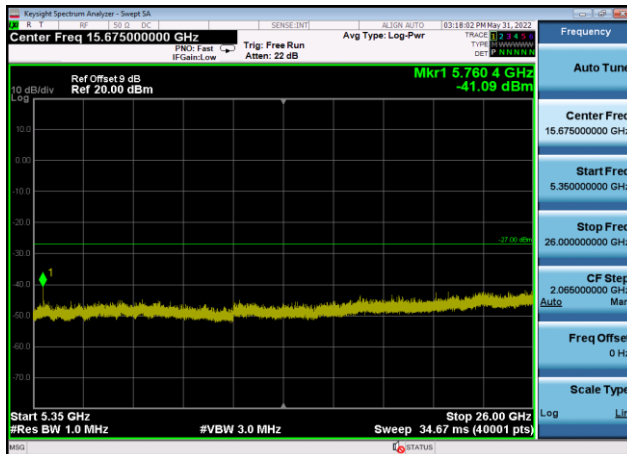
U-NII-1 ,Plot 3,5350MHz~26000MHz-802. 11a(20MHz),5220MHz,Ant9
