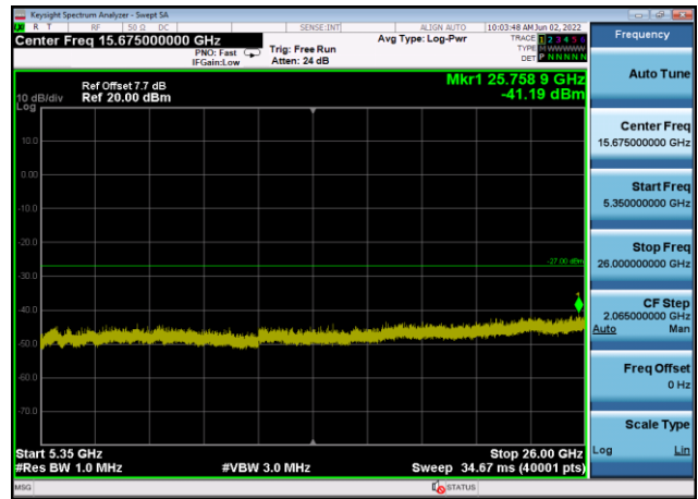
U-NII-1 ,Plot 3,5350MHz~26000MHz-802. 11ac(40MHz),5230MHz,Ant8
