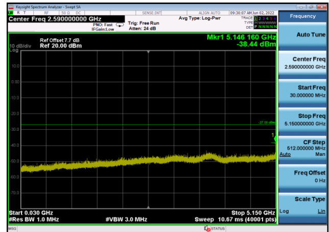
U-NII-1 ,Plot 2,30MHz~5150MHz-802.11a x(20MHz),5220MHz,Ant8
