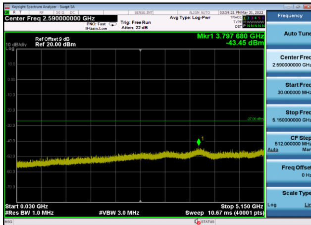
U-NII-1 ,Plot 2,30MHz~5150MHz-802.11a c(40MHz),5230MHz,Ant9
