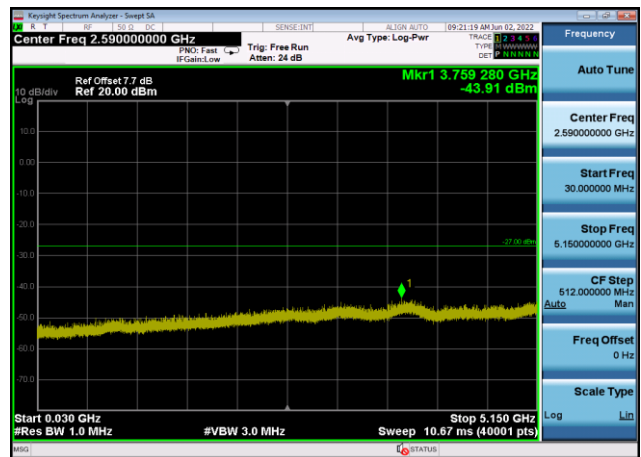
U-NII-1 ,Plot 2,30MHz~5150MHz-802.11a c(20MHz),5240MHz,Ant8
