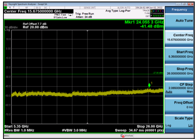
U-NII-1 ,Plot 3,5350MHz~26000MHz-802. 11ac(20MHz),5220MHz,Ant8
