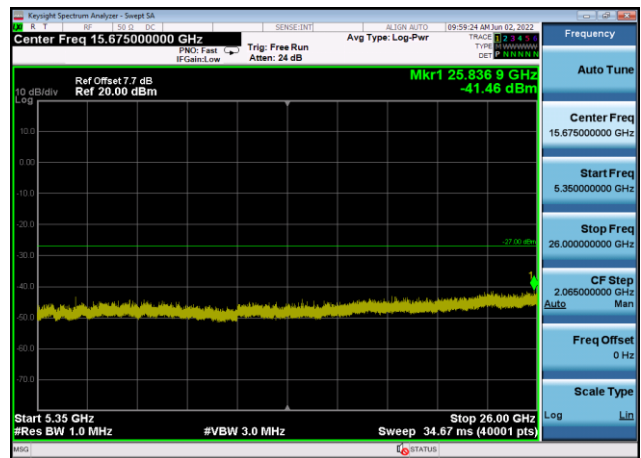
U-NII-1 ,Plot 3,5350MHz~26000MHz-802. 11ac(80MHz),5210MHz,Ant8
