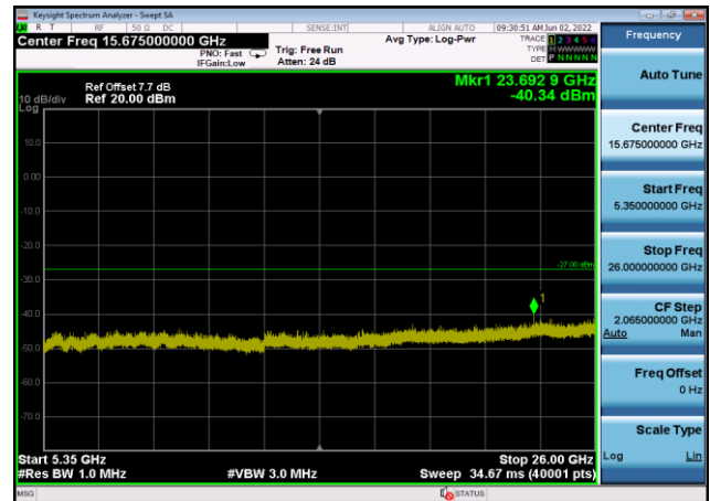
U-NII-1 ,Plot 3,5350MHz~26000MHz-802. 11ax(20MHz),5220MHz,Ant8
