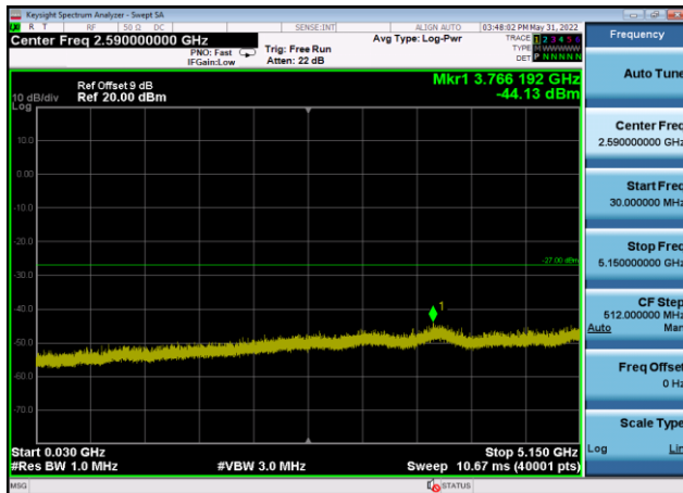
U-NII-1 ,Plot 2,30MHz~5150MHz-802.11a x(20MHz),5220MHz,Ant9
