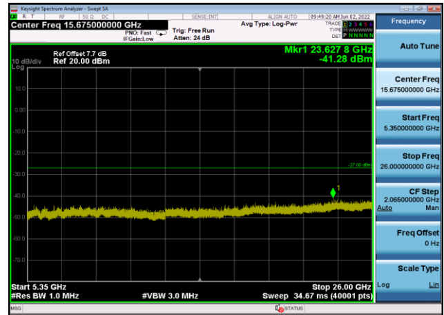
U-NII-1 ,Plot 3,5350MHz~26000MHz-802. 11ax(80MHz),5210MHz,Ant8
