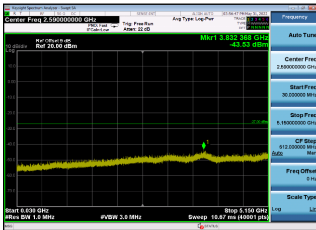
U-NII-1 ,Plot 2,30MHz~5150MHz-802.11a c(80MHz),5210MHz,Ant9
