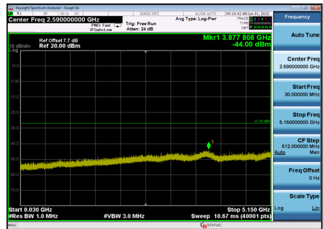
U-NII-1 ,Plot 2,30MHz~5150MHz-802.11a (20MHz),5240MHz,Ant8
