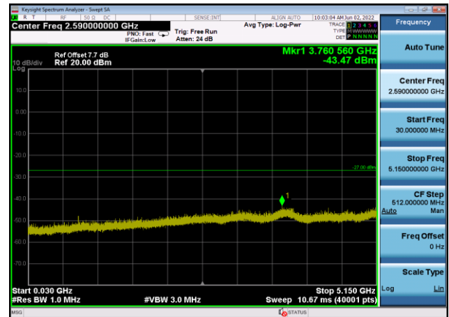
U-NII-1 ,Plot 2,30MHz~5150MHz-802.11a c(40MHz),5230MHz,Ant8
