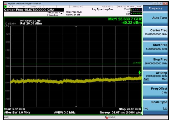
U-NII-1 ,Plot 3,5350MHz~26000MHz-802. 11ax(40MHz),5230MHz,Ant8
