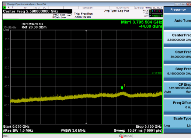
U-NII-1 ,Plot 2,30MHz~5150MHz-802.11a x(40MHz),5230MHz,Ant9
