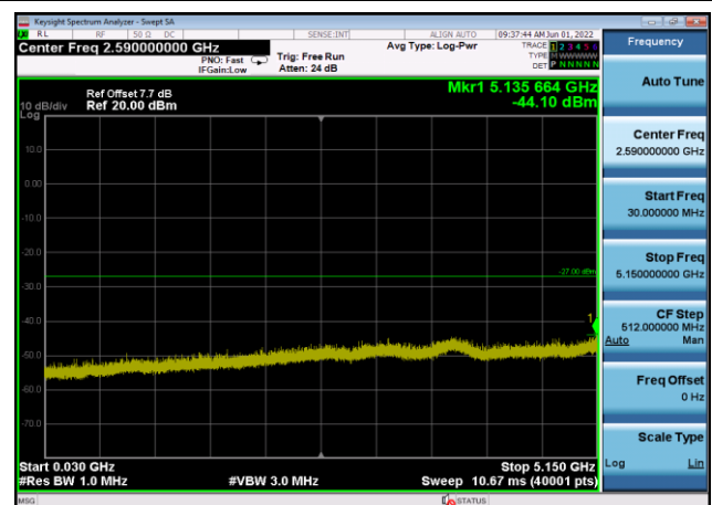
U-NII-2a ,Plot 2,30MHz~5150MHz-802.11 a(20MHz),5260MHz,Ant8
