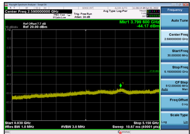
U-NII-2a ,Plot 2,30MHz~5150MHz-802.11 n(20MHz),5300MHz,Ant8
