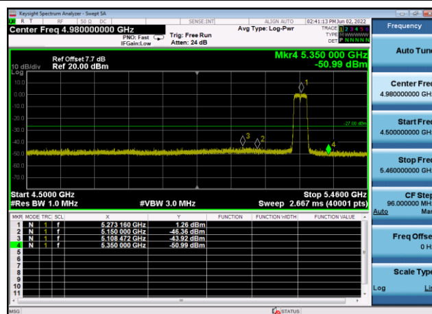
U-NII-2a ,Plot 1,Band Edge-802.11ac(4 0MHz),5310MHz,Ant8
