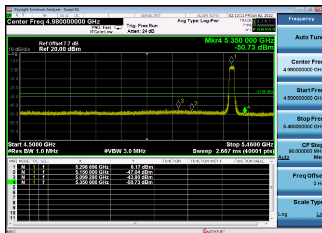
U-NII-2a ,Plot 1,Band Edge-802.11ax(2 0MHz),5320MHz,Ant8
