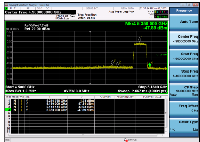
U-NII-2a ,Plot 1,Band Edge-802.11ax(1 60MHz),5250MHz,Ant8
