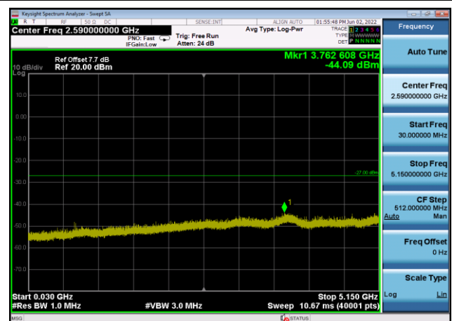
U-NII-2a ,Plot 2,30MHz~5150MHz-802.11 ac(20MHz),5320MHz,Ant8
