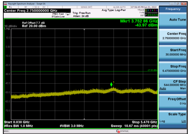
U-NII-2c ,Plot 2,30MHz~5470MHz-802.11 n(40MHz),5670MHz,Ant8
