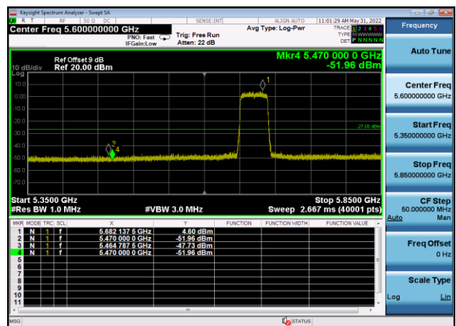
U-NII-2c ,Plot 1,Band Edge-802.11ax(4 0MHz),5670MHz,Ant9
