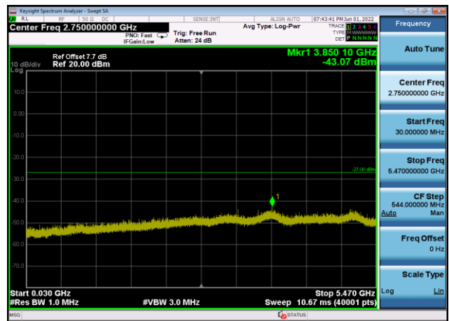
U-NII-2c ,Plot 2,30MHz~5470MHz-802.11 ac(40MHz),5670MHz,Ant8
