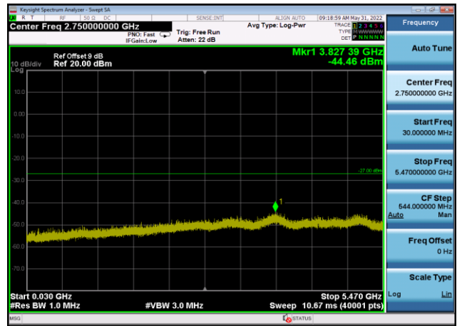
U-NII-2c ,Plot 2,30MHz~5470MHz-802.11 a(20MHz),5700MHz,Ant9
