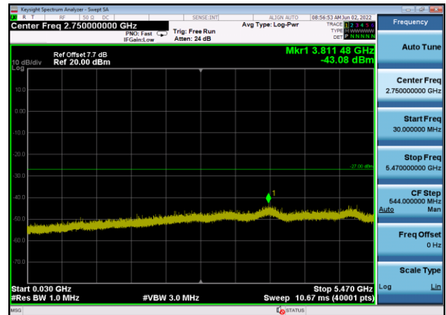
U-NII-2c ,Plot 2,30MHz~5470MHz-802.11 ax(20MHz),5600MHz,Ant8
