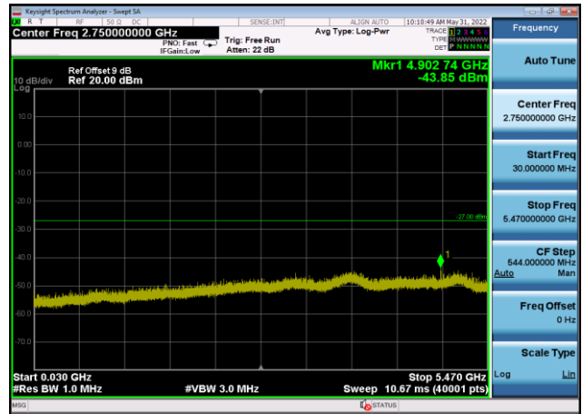
U-NII-2c ,Plot 2,30MHz~5470MHz-802.11 ac(20MHz),5700MHz,Ant8
