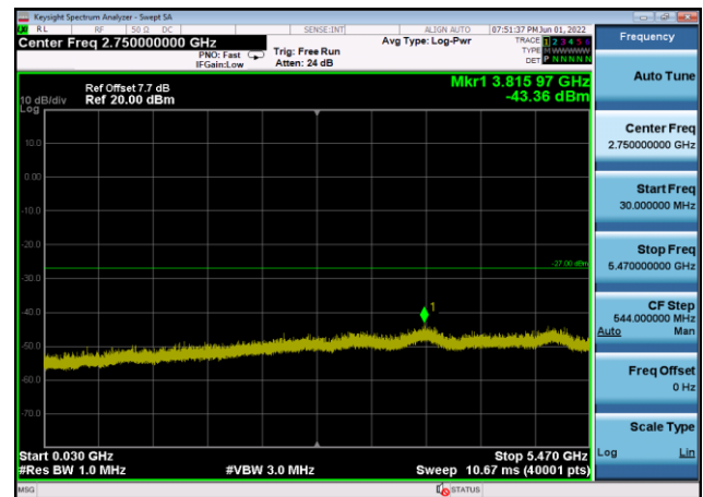
U-NII-2c ,Plot 2,30MHz~5470MHz-802.11 ax(40MHz),5590MHz,Ant8
