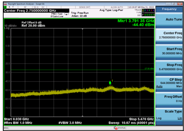
U-NII-2c ,Plot 2,30MHz~5470MHz-802.11 ac(20MHz),5600MHz,Ant9
