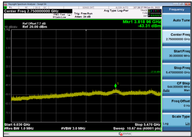
U-NII-2c ,Plot 2,30MHz~5470MHz-802.11 ac(40MHz),5590MHz,Ant8
