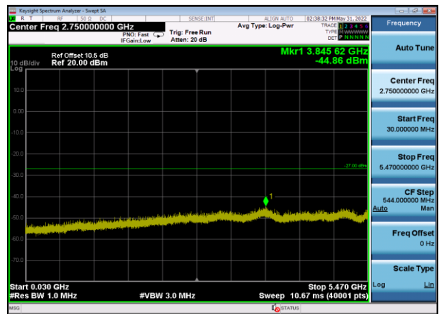
U-NII-2c ,Plot 2,30MHz~5470MHz-802.11 ac(160MHz),5570MHz,Ant9
