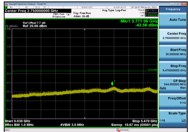
U-NII-2c ,Plot 2,30MHz~5470MHz-802.11 ax(80MHz),5610MHz,Ant8
