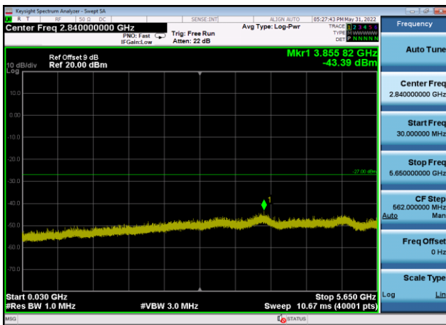
U-NII-3 ,Plot 2,30MHz~5650MHz-802.11n (20MHz),5825MHz,Ant9
