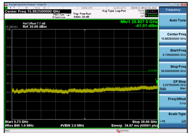
U-NII-2c ,Plot 3,5725MHz~26000MHz-802 .11ac(160MHz),5570MHz,Ant8
