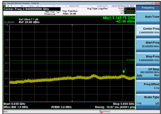
U-NII-3 ,Plot 2,30MHz~5650MHz-802.11n (20MHz),5825MHz,Ant8
