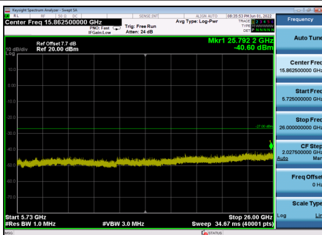
U-NII-2c ,Plot 3,5725MHz~26000MHz-802 .11ac(20MHz),5700MHz,Ant8
