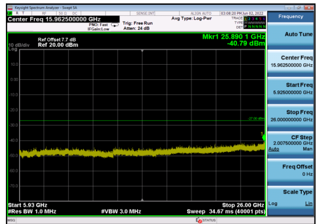
U-NII-3 ,Plot 3,5925MHz~26000MHz-802. 11n(20MHz),5825MHz,Ant8
