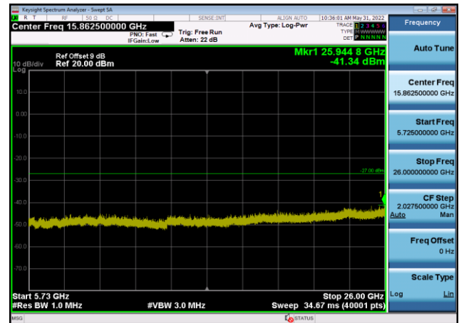
U-NII-2c ,Plot 3,5725MHz~26000MHz-802 .11ax(20MHz),5700MHz,Ant9
