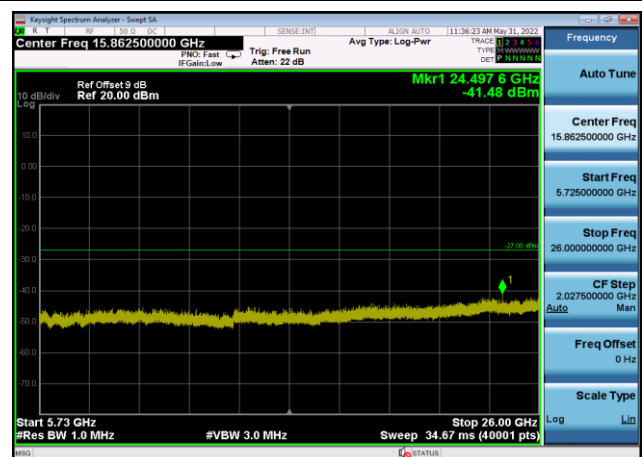
U-NII-2c ,Plot 3,5725MHz~26000MHz-802 .11ac(40MHz),5510MHz,Ant9
