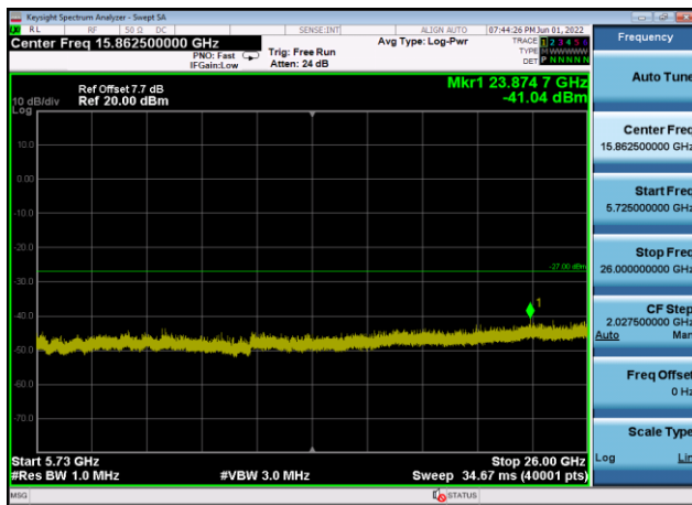
U-NII-2c ,Plot 3,5725MHz~26000MHz-802 .11ac(40MHz),5670MHz,Ant8
