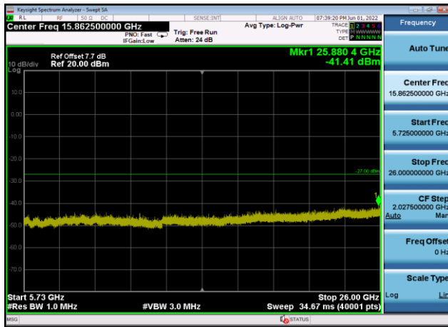
U-NII-2c ,Plot 3,5725MHz~26000MHz-802 .11ac(40MHz),5590MHz,Ant8
