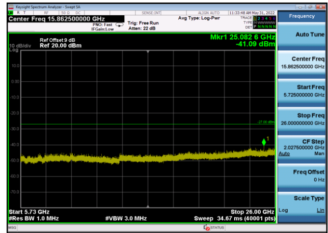
U-NII-2c ,Plot 3,5725MHz~26000MHz-802 .11ac(40MHz),5670MHz,Ant9
