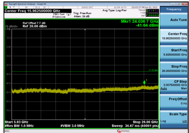
U-NII-3 ,Plot 3,5925MHz~26000MHz-802. 11n(20MHz),5785MHz,Ant8
