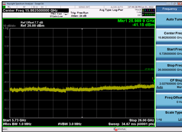
U-NII-2c ,Plot 3,5725MHz~26000MHz-802 .11ax(40MHz),5670MHz,Ant8
