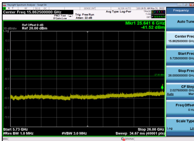
U-NII-2c ,Plot 3,5725MHz~26000MHz-802 .11ac(20MHz),5600MHz,Ant9
