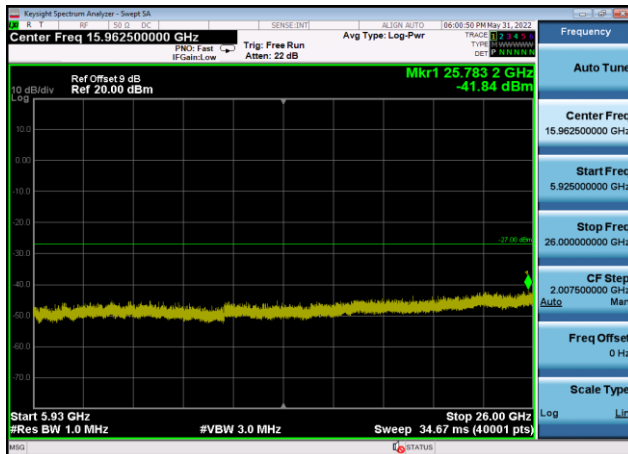
U-NII-3 ,Plot 3,5925MHz~26000MHz-802. 11n(20MHz),5785MHz,Ant9
