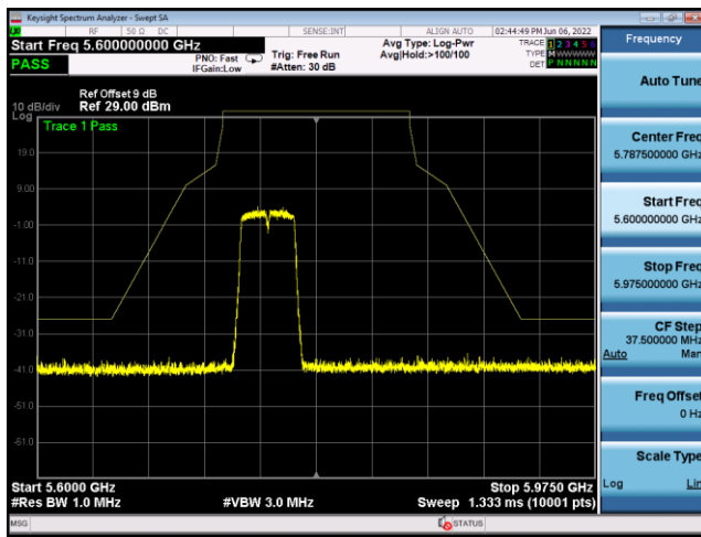
U-NII-3 ,Plot 1,Band Edge-802.11ac(40 MHz),5795MHz,Ant9
