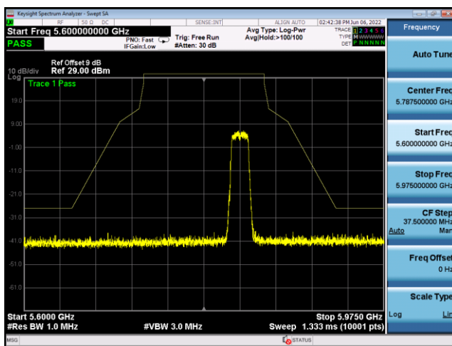
U-NII-3 ,Plot 1,Band Edge-802.11ac(20 MHz),5825MHz,Ant9
