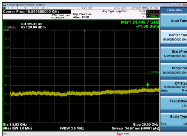
U-NII-3 ,Plot 3,5925MHz~26000MHz-802.11n(40MHz),5795MHz,Ant9
