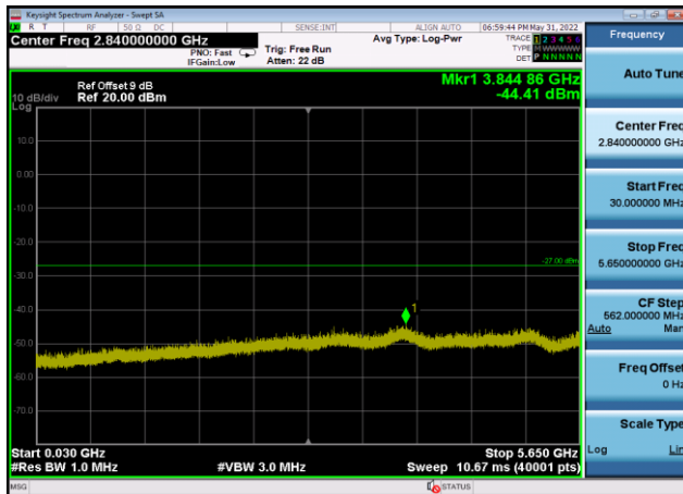
U-NII-3 ,Plot 2,30MHz~5650MHz-802.11a c(40MHz),5795MHz,Ant9
