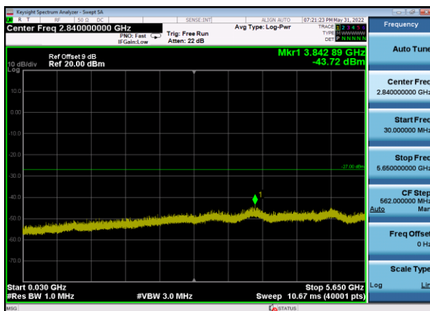
U-NII-3 ,Plot 2,30MHz~5650MHz-802.11a c(80MHz),5775MHz,Ant9
