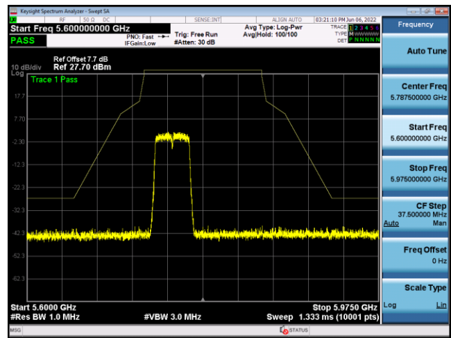
U-NII-3 ,Plot 1,Band Edge-802.11ac(40 MHz),5795MHz,Ant8
