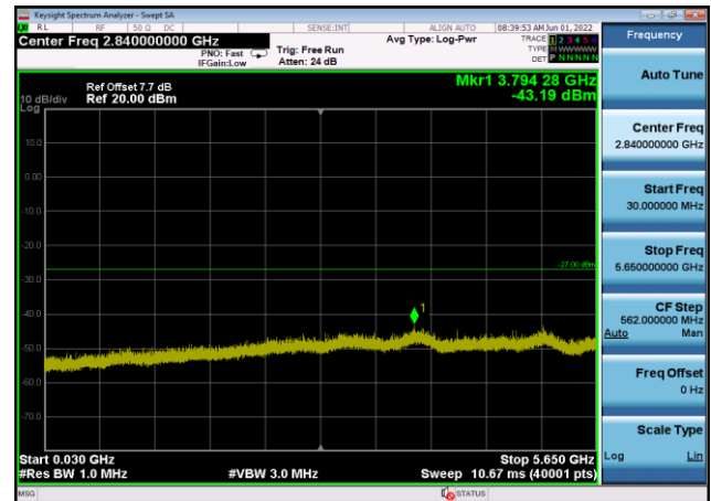
U-NII-3 ,Plot 2,30MHz~5650MHz-802.11a (20MHz),5785MHz,Ant8
