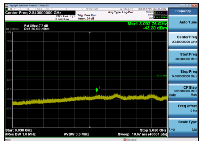
U-NII-3 ,Plot 2,30MHz~5650MHz-802.11a c(80MHz),5775MHz,Ant8
