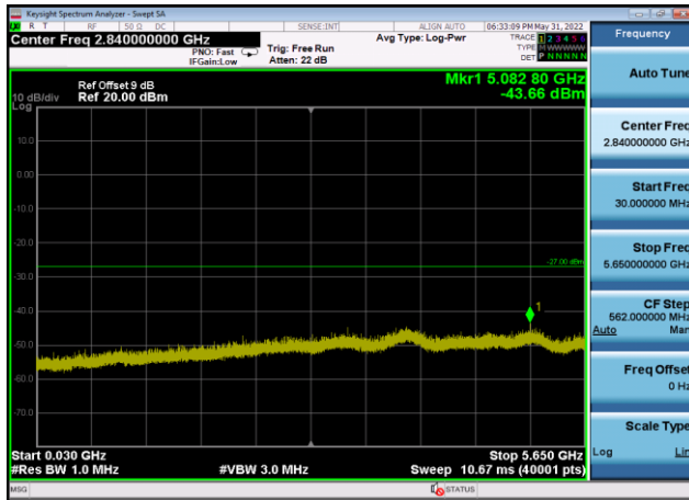
U-NII-3 ,Plot 2,30MHz~5650MHz-802.11a x(20MHz),5825MHz,Ant9
