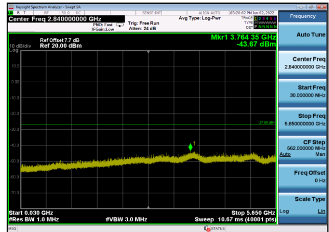
U-NII-3 ,Plot 2,30MHz~5650MHz-802.11a c(40MHz),5795MHz,Ant8
