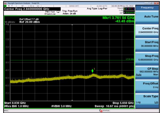
U-NII-3 ,Plot 2,30MHz~5650MHz-802.11a x(20MHz),5825MHz,Ant8
