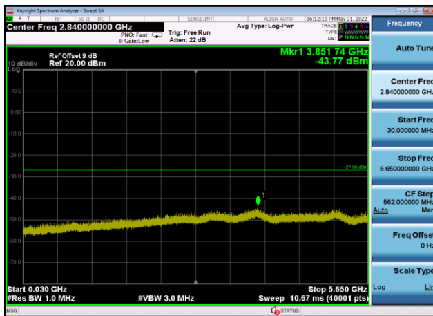
U-NII-3 ,Plot 2,30MHz~5650MHz-802.11a c(20MHz),5825MHz,Ant9
