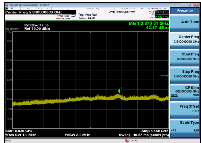
U-NII-3 ,Plot 2,30MHz~5650MHz-802.11a (20MHz),5825MHz,Ant8
