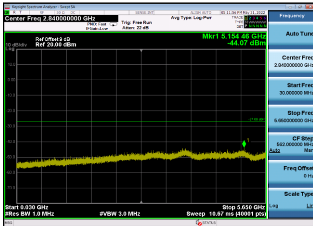
U-NII-3 ,Plot 2,30MHz~5650MHz-802.11a (20MHz),5785MHz,Ant9
