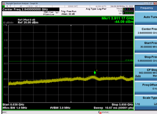
U-NII-3 ,Plot 2,30MHz~5650MHz-802.11a c(20MHz),5785MHz,Ant9
