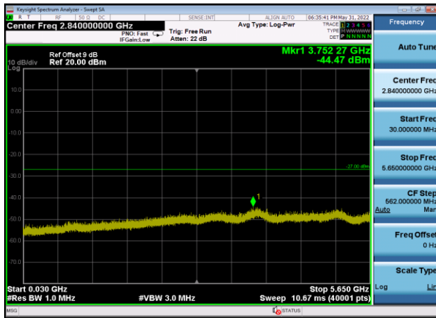
U-NII-3 ,Plot 2,30MHz~5650MHz-802.11a x(20MHz),5785MHz,Ant9
