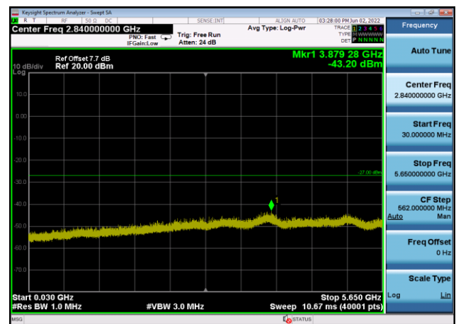
U-NII-3 ,Plot 2,30MHz~5650MHz-802.11a c(20MHz),5825MHz,Ant8
