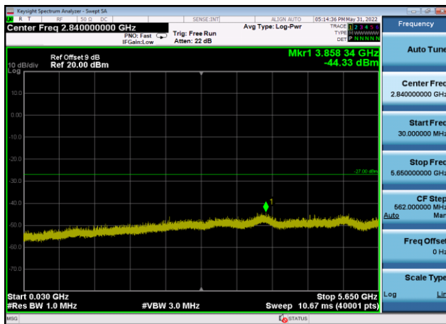
U-NII-3 ,Plot 2,30MHz~5650MHz-802.11a (20MHz),5825MHz,Ant9
