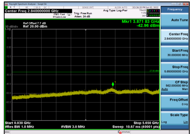
U-NII-3 ,Plot 2,30MHz~5650MHz-802.11a c(20MHz),5785MHz,Ant8
