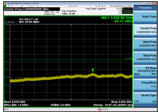
U-NII-3 ,Plot 2,30MHz~5650MHz-802.11a x(20MHz),5785MHz,Ant8
