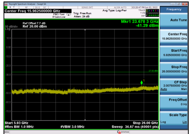
U-NII-3 ,Plot 3,5925MHz~26000MHz-802. 11ac(40MHz),5795MHz,Ant8
