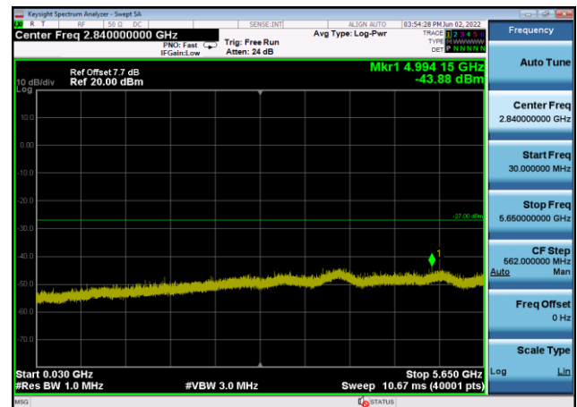
U-NII-3 ,Plot 2,30MHz~5650MHz-802.11a x(80MHz),5775MHz,Ant8
