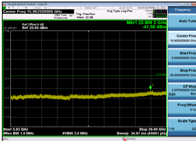
U-NII-3 ,Plot 3,5925MHz~26000MHz-802. 11ax(40MHz),5795MHz,Ant9
