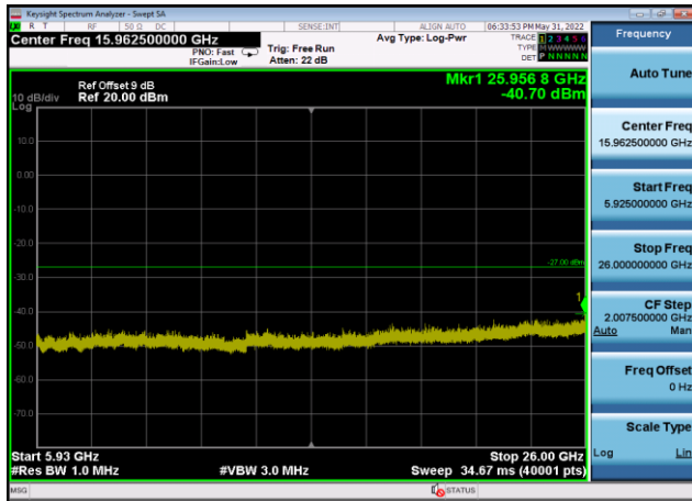
U-NII-3 ,Plot 3,5925MHz~26000MHz-802. 11ax(20MHz),5825MHz,Ant9
