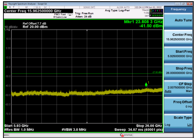
U-NII-3 ,Plot 3,5925MHz~26000MHz-802. 11ac(20MHz),5825MHz,Ant8
