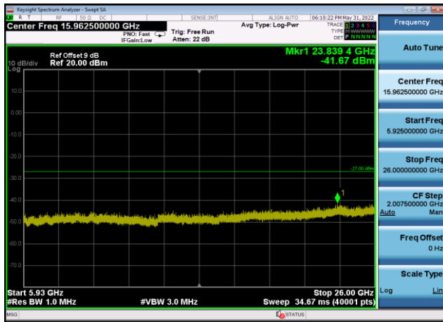
U-NII-3 ,Plot 3,5925MHz~26000MHz-802. 11ac(20MHz),5785MHz,Ant9
