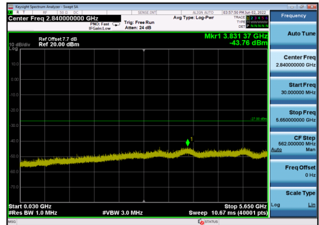
U-NII-3 ,Plot 2,30MHz~5650MHz-802.11a x(40MHz),5795MHz,Ant8
