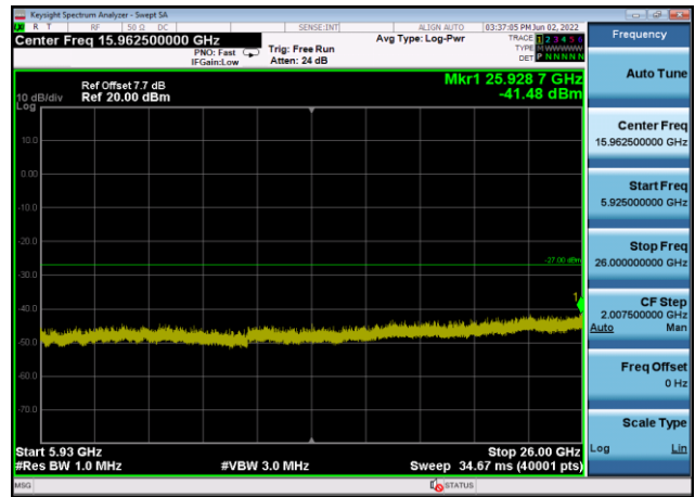
U-NII-3 ,Plot 3,5925MHz~26000MHz-802. 11ac(20MHz),5785MHz,Ant8
