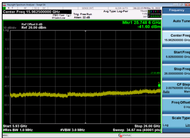
U-NII-3 ,Plot 3,5925MHz~26000MHz-802. 11ac(20MHz),5825MHz,Ant9
