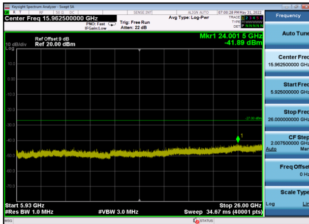
U-NII-3 ,Plot 3,5925MHz~26000MHz-802. 11ac(40MHz),5795MHz,Ant9
