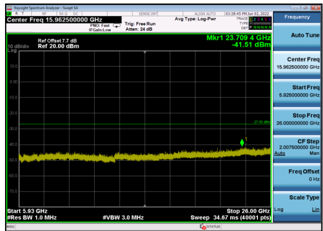
U-NII-3 ,Plot 3,5925MHz~26000MHz-802. 11ac(20MHz),5825MHz,Ant8
