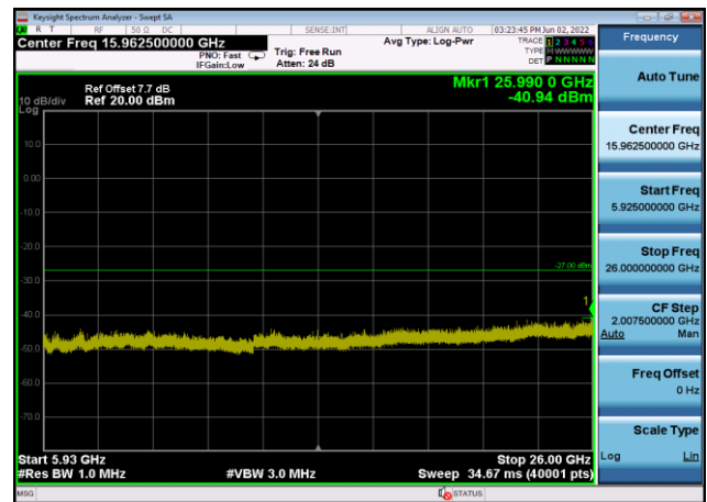
U-NII-3 ,Plot 3,5925MHz~26000MHz-802. 11ac(80MHz),5775MHz,Ant8
