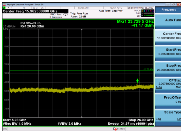
U-NII-3 ,Plot 3,5925MHz~26000MHz-802. 11ac(80MHz),5775MHz,Ant9
