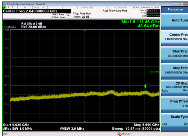
U-NII-3 ,Plot 2,30MHz~5650MHz-802.11a x(40MHz),5795MHz,Ant9
