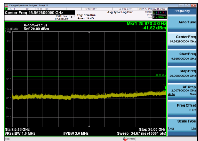
U-NII-3 ,Plot 3,5925MHz~26000MHz-802. 11ac(80MHz),5775MHz,Ant8
