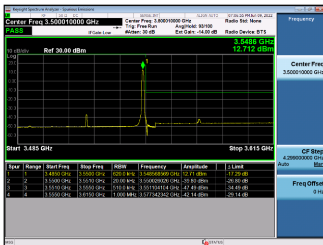
N77(80M)_DFT-s-OFDM_PI/2-BPSK_Edge_ 1RB_Left_Low_CH
