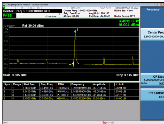
N77(60M)_CP-OFDM_QPSK_Edge_ 1RB_Left_Low_CH
