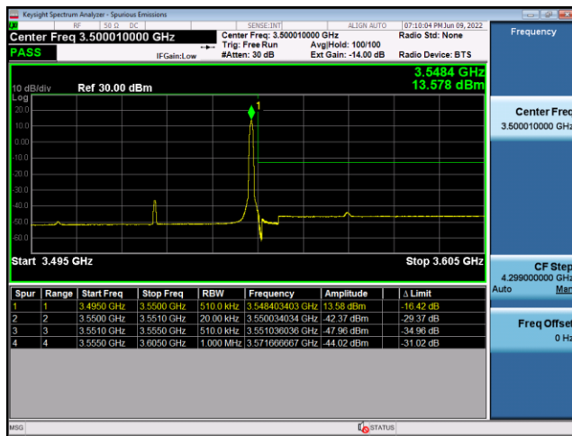
N77(60M)_DFT-s-OFDM_PI/2-BPSK_Edge_ 1RB_Left_Low_CH
