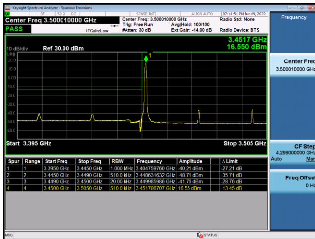
N77(50M)_CP-OFDM_QPSK_Edge_ 1RB_Left_Low_CH
