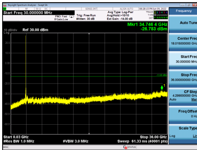
N77(90M)_DFT-s-OFDM_BPSK_ Edge_1RB_Left_Mid_CH
