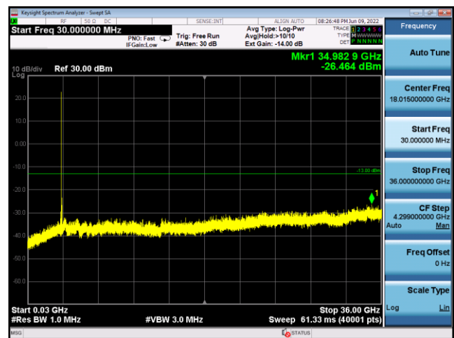
N77(90M)_CP-OFDM_QPSK_ Edge_1RB_Left_High_CH
