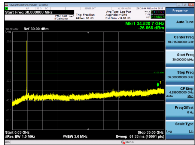
N77(90M)_CP-OFDM_QPSK_ Edge_1RB_Left_Mid_CH
