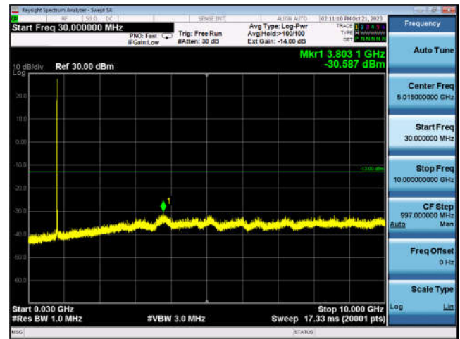
N41_100MHz_DFT-s-OFDM_BPSK_ Edge_1RB_Left_Low_CH
