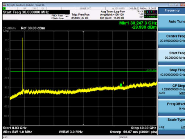
N78_80MHz_DFT-s-OFDM_BPSK_ Edge_1RB_Left_Low_CH
