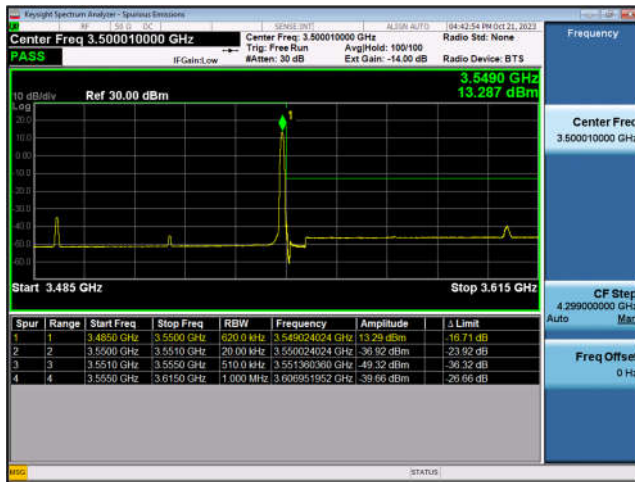
N78_80MHz_DFT-s-OFDM_PI/2-BPSK_Edge_ 1RB_Left_Low_CH
