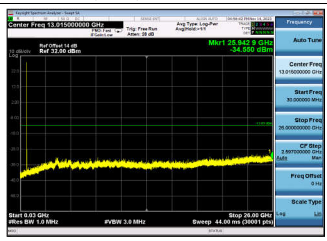
FDD17_HighRange_10MHz_30MHz~26GHz
