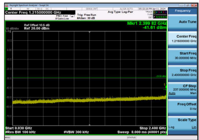
,Plot 3,30MHz~2400MHz-802.11n(40MHz) ,2437MHz,Ant12
