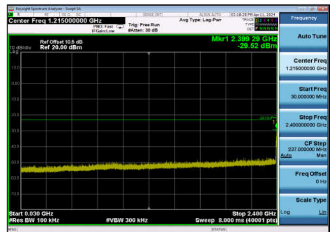
,Plot 3,30MHz~2400MHz-802.11n(20MHz) ,2437MHz,Ant12
