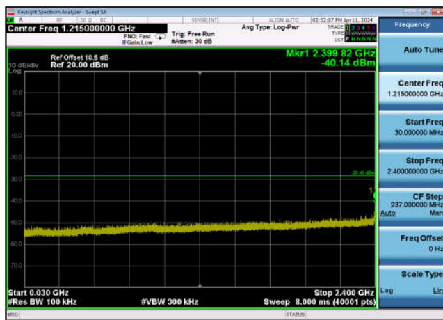
,Plot 3,30MHz~2400MHz-802.11n(40MHz) ,2437MHz,Ant13
