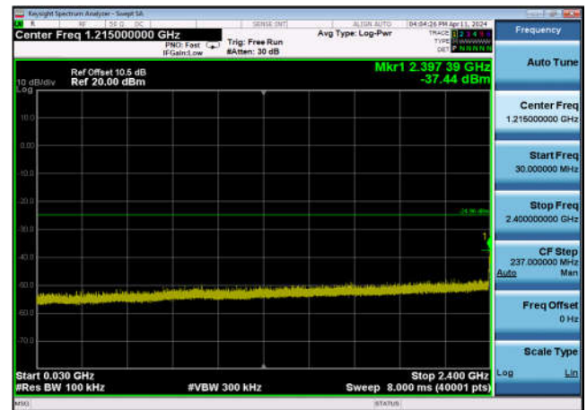
,Plot 3,30MHz~2400MHz-802.11ax(20MHz) ,2437MHz,Ant12
