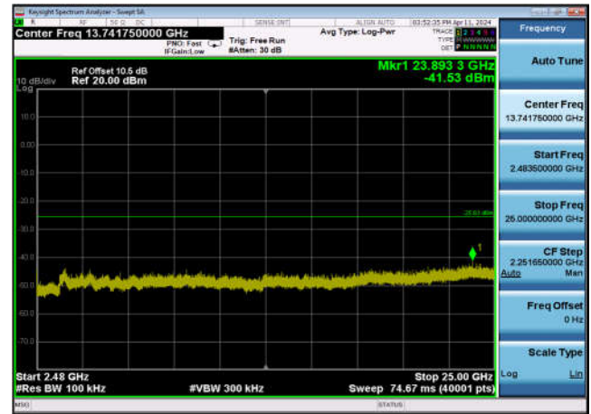
,Plot 4,2483.5MHz~25000MHz-802.11ax(4 0MHz),2422MHz,Ant12
