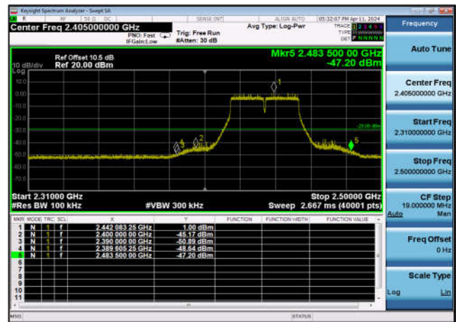
,Plot 2,Band Edge-802.11n(40MHz) ,2437MHz,Ant12
