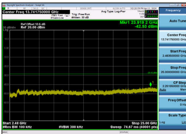
,Plot 4,2483.5MHz~25000MHz-802.11ax(4 0MHz),2437MHz,Ant13
