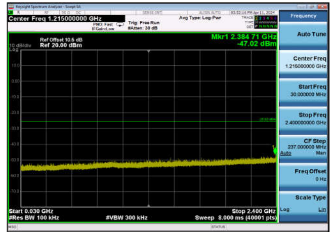
,Plot 3,30MHz~2400MHz-802.11ax(40MHz) ,2422MHz,Ant12
