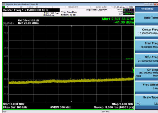
,Plot 3,30MHz~2400MHz-802.11n(20MHz) ,2437MHz,Ant13
