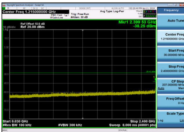
,Plot 3,30MHz~2400MHz-802.11ax(40MHz) ,2437MHz,Ant13
