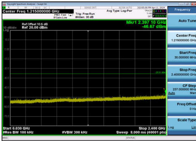
,Plot 3,30MHz~2400MHz-802.11ax(40MHz) ,2422MHz,Ant13
