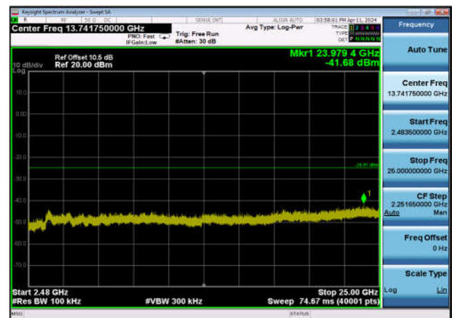
,Plot 4,2483.5MHz~25000MHz-802.11ax(2 0MHz),2437MHz,Ant12
