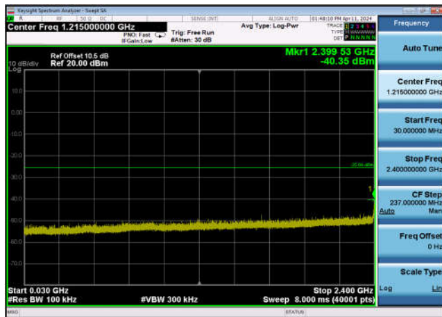
,Plot 3,30MHz~2400MHz-802.11ax(20MHz) ,2437MHz,Ant13
