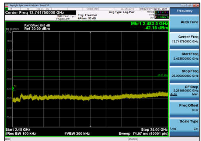
,Plot 4,2483.5MHz~25000MHz-802.11ax(4 0MHz),2437MHz,Ant12
