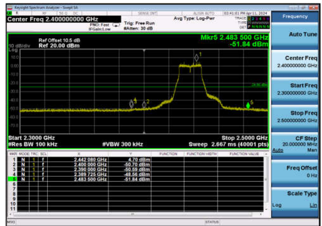
,Plot 2,Band Edge-802.11n(20MHz) ,2437MHz,Ant12
