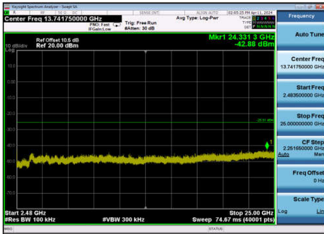
,Plot 4,2483.5MHz~25000MHz-802.11ax(4 0MHz),2422MHz,Ant13
