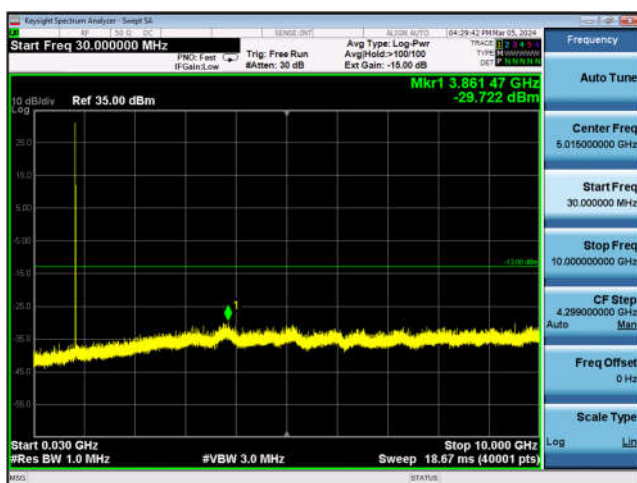
GSM 850-251, 30MHz ~10GHz
