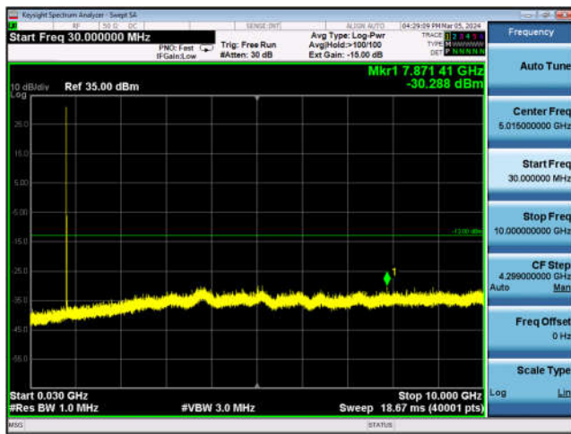
GSM 850-190, 30MHz ~10GHz
