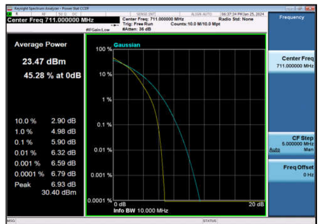
FDD17_HighRange_10MHz_711_fullRB _Q16
