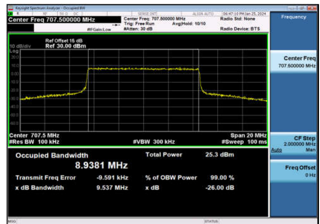
FDD12_MidRange_10_707.5_Q16
