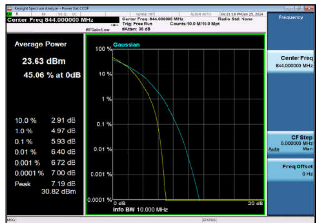
FDD05_HighRange_10MHz_844_fullRB _Q16
