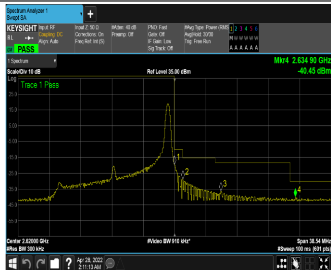
Band38-15MHz-QPSK-38175-1RB#74
