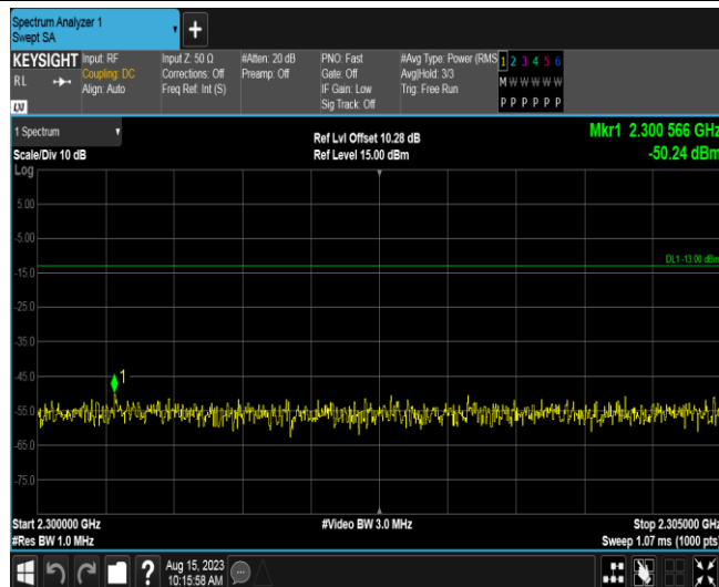
Band40-10MHz-QPSK-38750-1RB#0-Range6:2300~2305MHz
