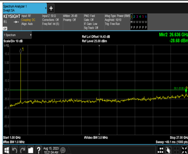
Band41-5MHz-QPSK-40620-1RB#0-Range2:1000~27000MHz
