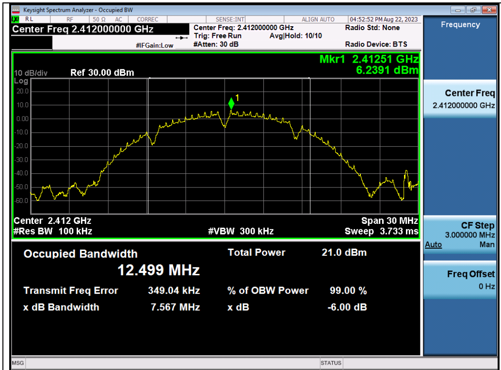
Test_Graph_802.11b_ANT1_2412_1Mbps_DTBSW
