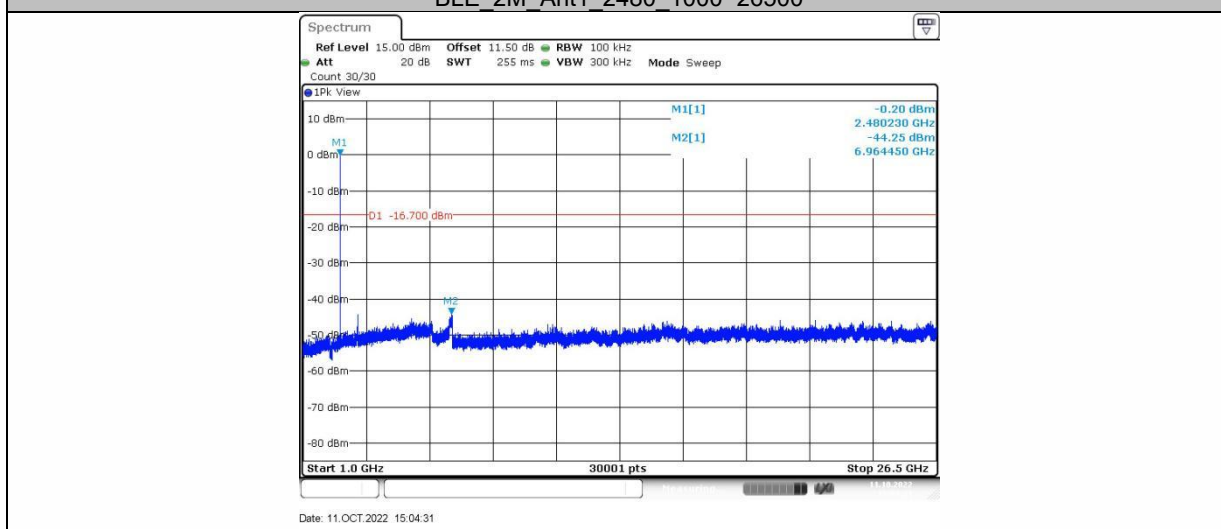
BLE_2M_Ant1_2480_1000~26500
