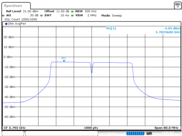
802.11ac40_5795MHz
