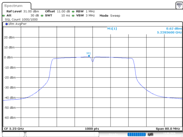
802.11ac40_5230MHz
