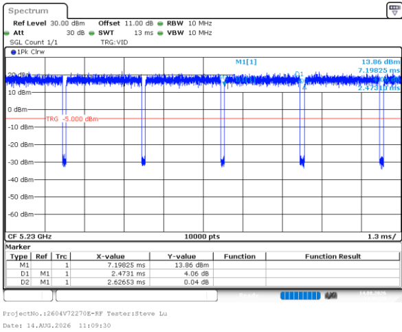
802.11ac40_5230MHz
