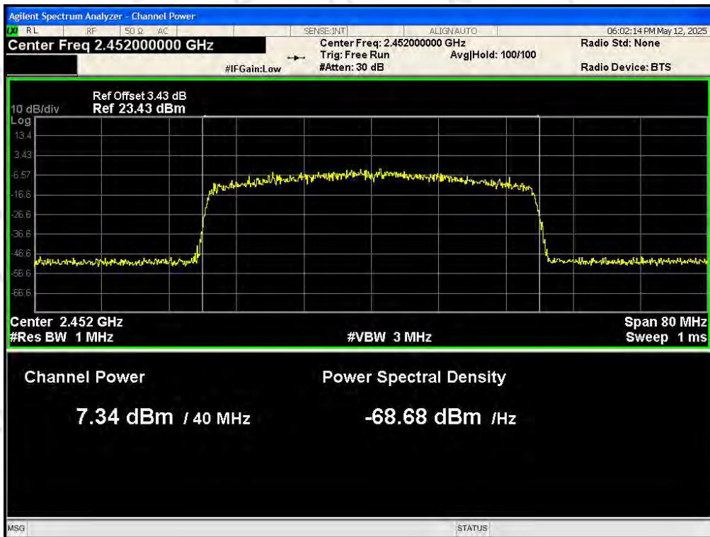
Power NVNT 802.11ax40 2452MHz Ant0
