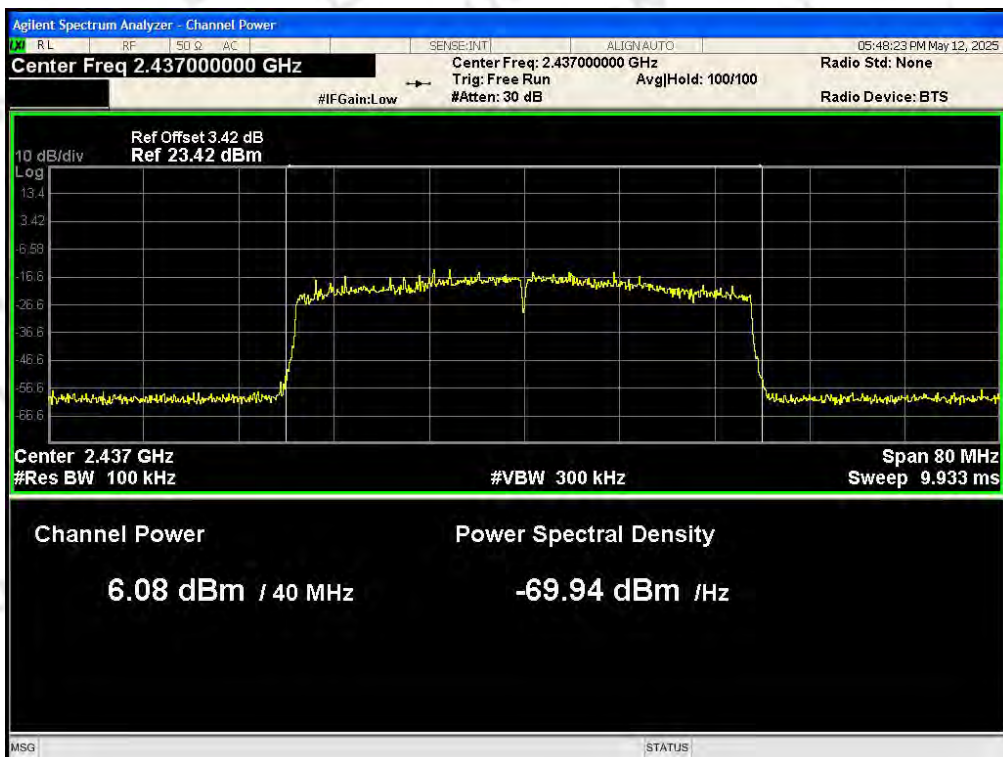
Power NVNT 802.11ax40 2437MHz Ant0
