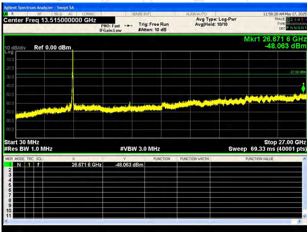
Tx. Spurious MIMO 802.11ac40 5310MHz Ant0&amp;1 Emission
