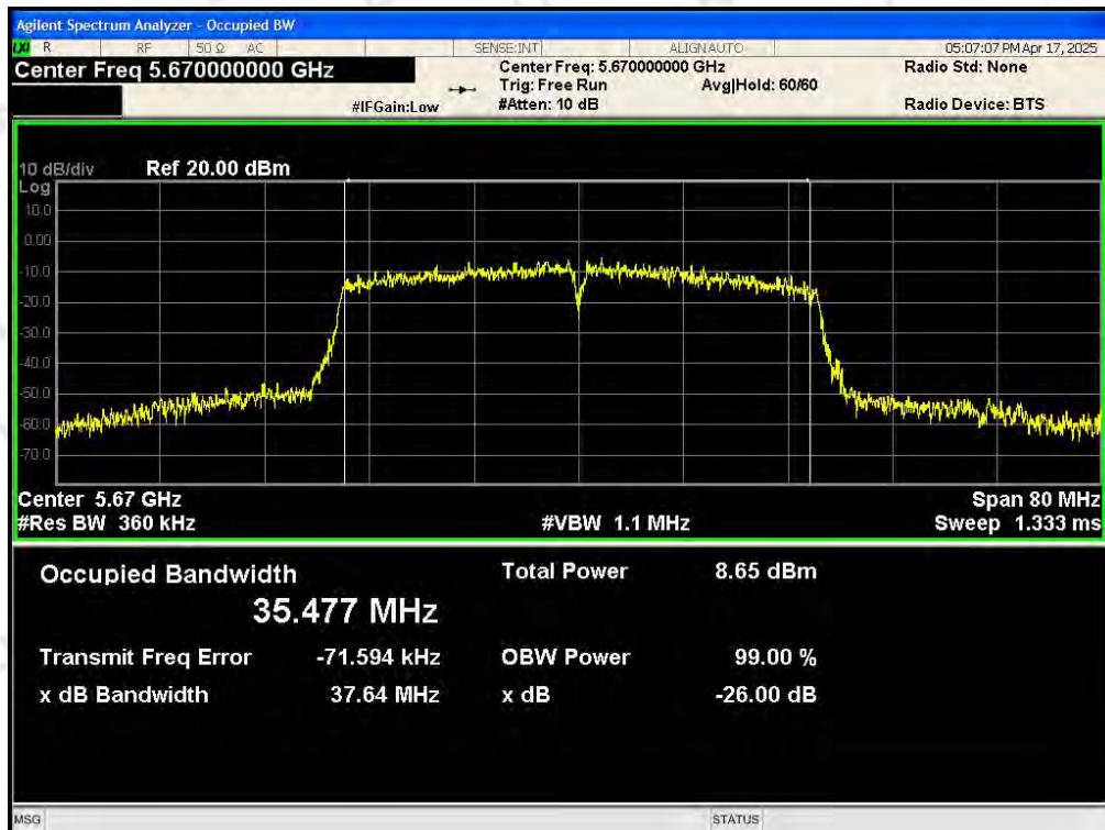
OBW NVNT 802.11ac40 5670MHz Ant0
