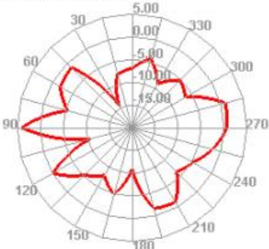
5450.000MHz E1
