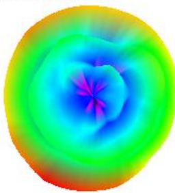
5100.000MHz
