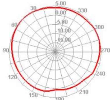
5450.000MHz H
