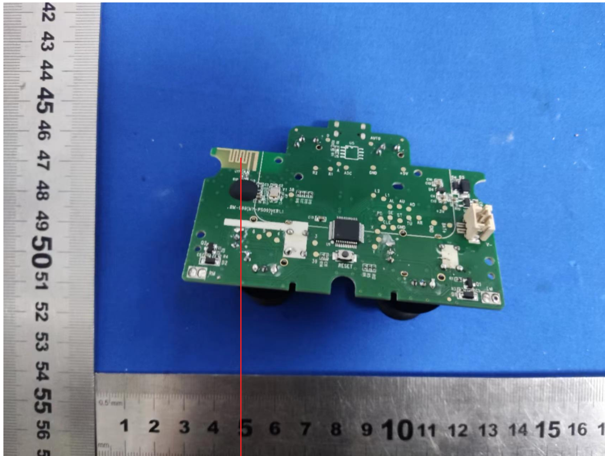
PCB ANT
