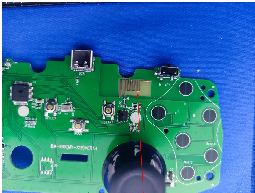
PCB ANT
