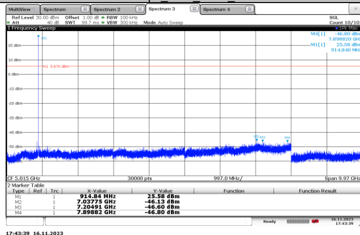
2GFSK-25 kbps Ant1 MCH_Spurious
