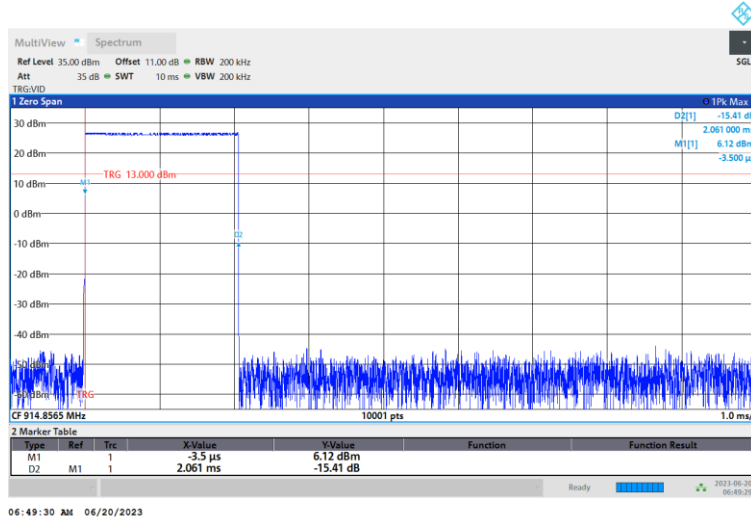
2GFSK-150 kbps _Ant1_Hop- BurstWidth 2
