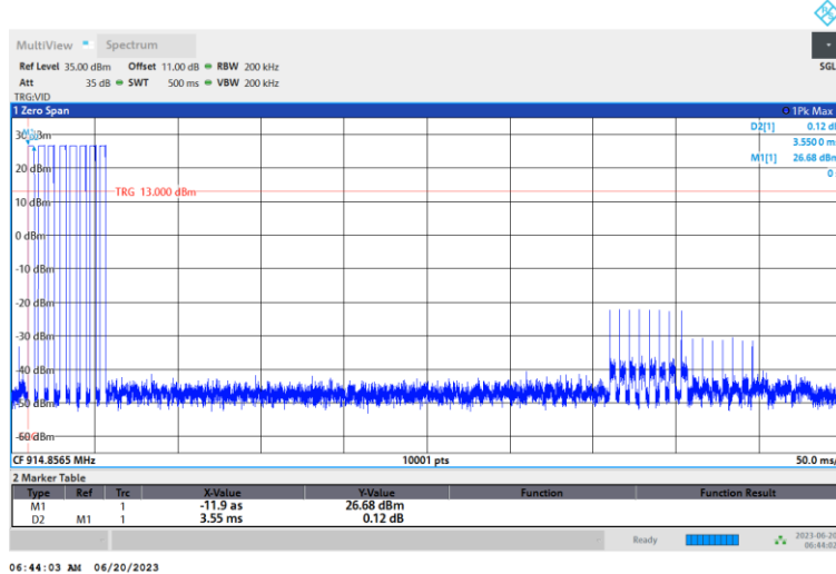
2GFSK-150 kbps _Ant1_Hop- BurstWidth 1
