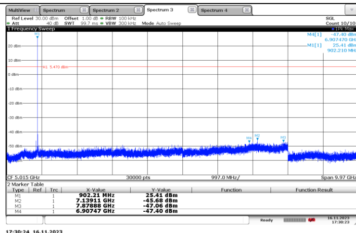
2GFSK-25 kbps Ant1 LCH_Spurious
