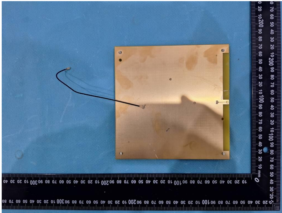
UHF ANT
