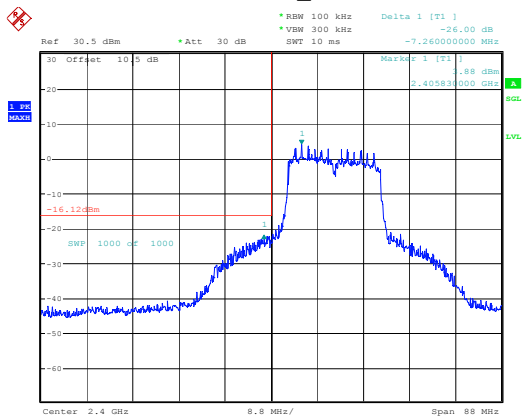
802.11n20_2412MHz
