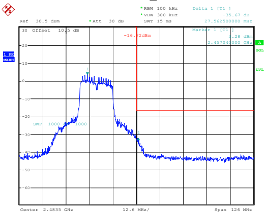
802.11n20_2462MHz
