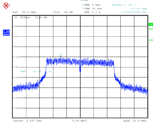
802.11g_2437MHz
