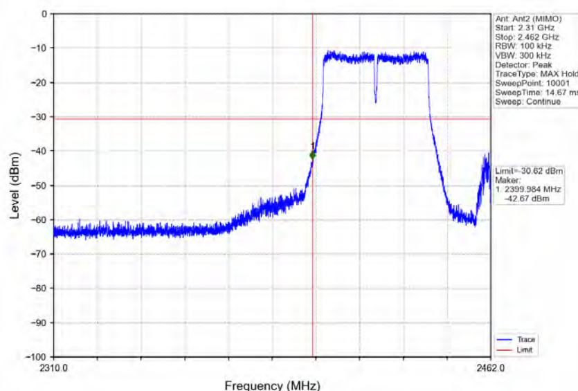
802.11n(HT40)_LCH_2422MHz_Ant2 (MIMO)_NTNV
