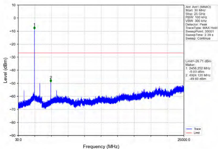
802.11n(HT20)_HCH_2462MHz_Ant1 (MIMO)_NTNV
