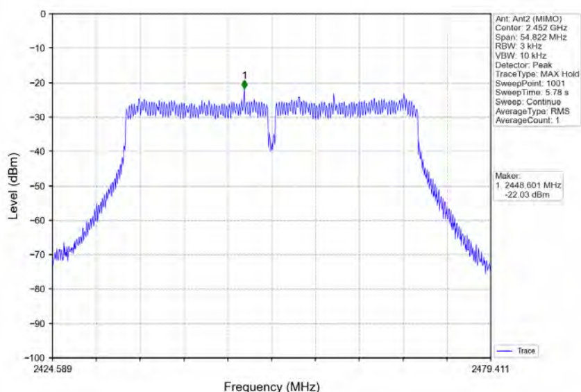
802.11n(HT40)_HCH_2452MHz_MIMO_NTNV
