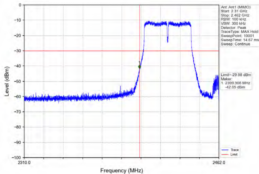
802.11n(HT40)_LCH_2422MHz_Ant1 (MIMO)_NTNV
