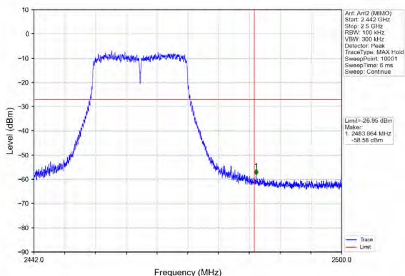
802.11n(HT20)_HCH_2462MHz_Ant2 (MIMO)_NTNV
