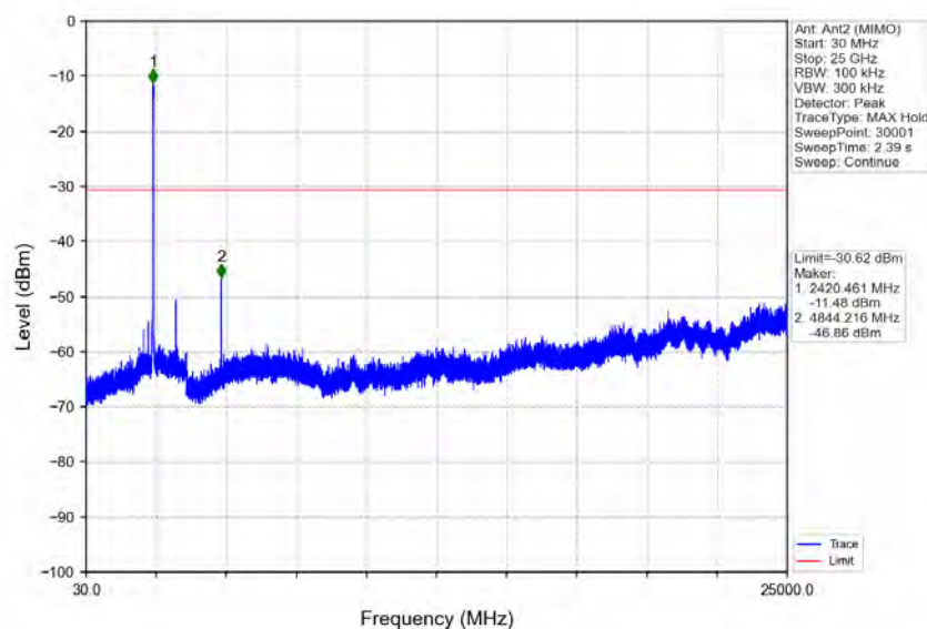
802.11n(HT40)_LCH_2422MHz_Ant2 (MIMO)_NTNV
