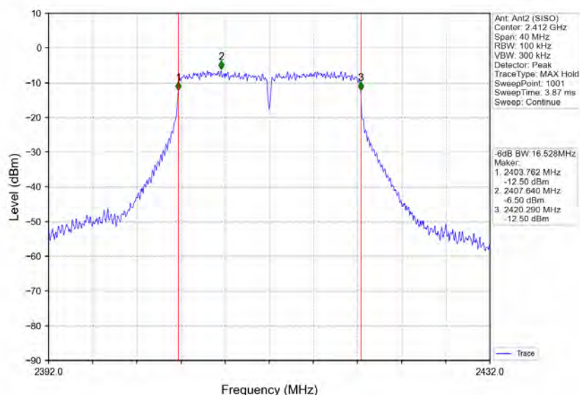
802.11g_LCH_2412MHz_Ant2 (SISO)_NTNV
