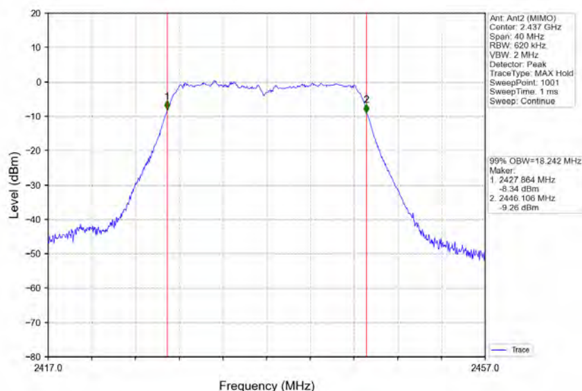
802.11n(HT20)_MCH_2437MHz_Ant2 (MIMO)_NTNV
