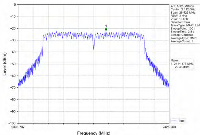
802.11n(HT20)_LCH_2412MHz_Ant2 (MIMO)_NTNV
