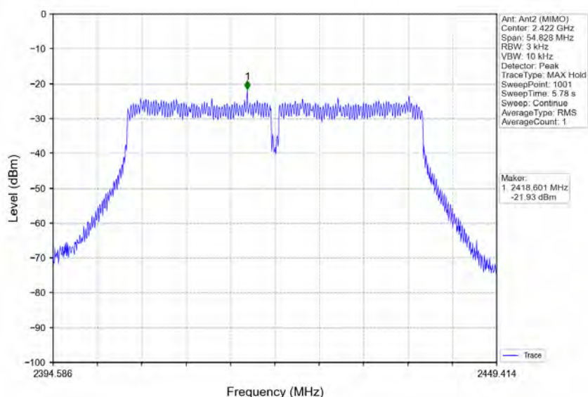
802.11n(HT40)_LCH_2422MHz_MIMO_NTNV
