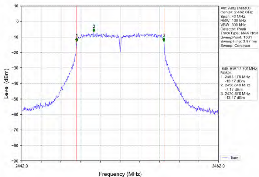
802.11n(HT20)_HCH_2462MHz_Ant2 (MIMO)_NTNV
