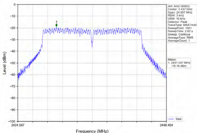
802.11g_MCH_2437MHz_Ant2 (SISO)_NTNV
