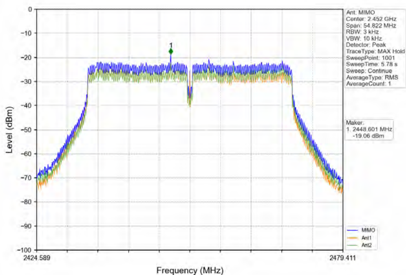
802.11n(HT40)_HCH_2452MHz_MIMO_NTNV
