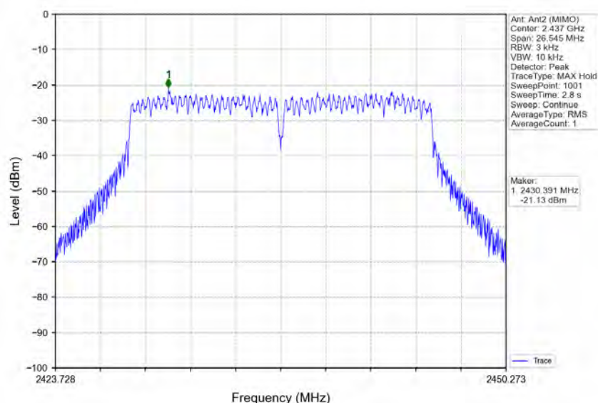
802.11n(HT20)_MCH_2437MHz_MIMO _NTNV
