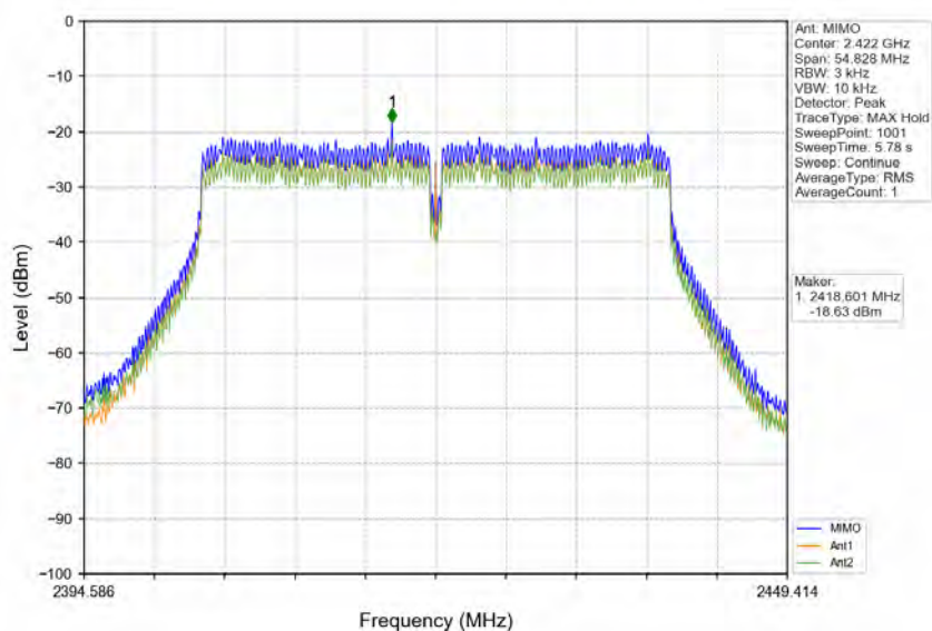
802.11n(HT40)_LCH_2422MHz_MIMO_NTNV
