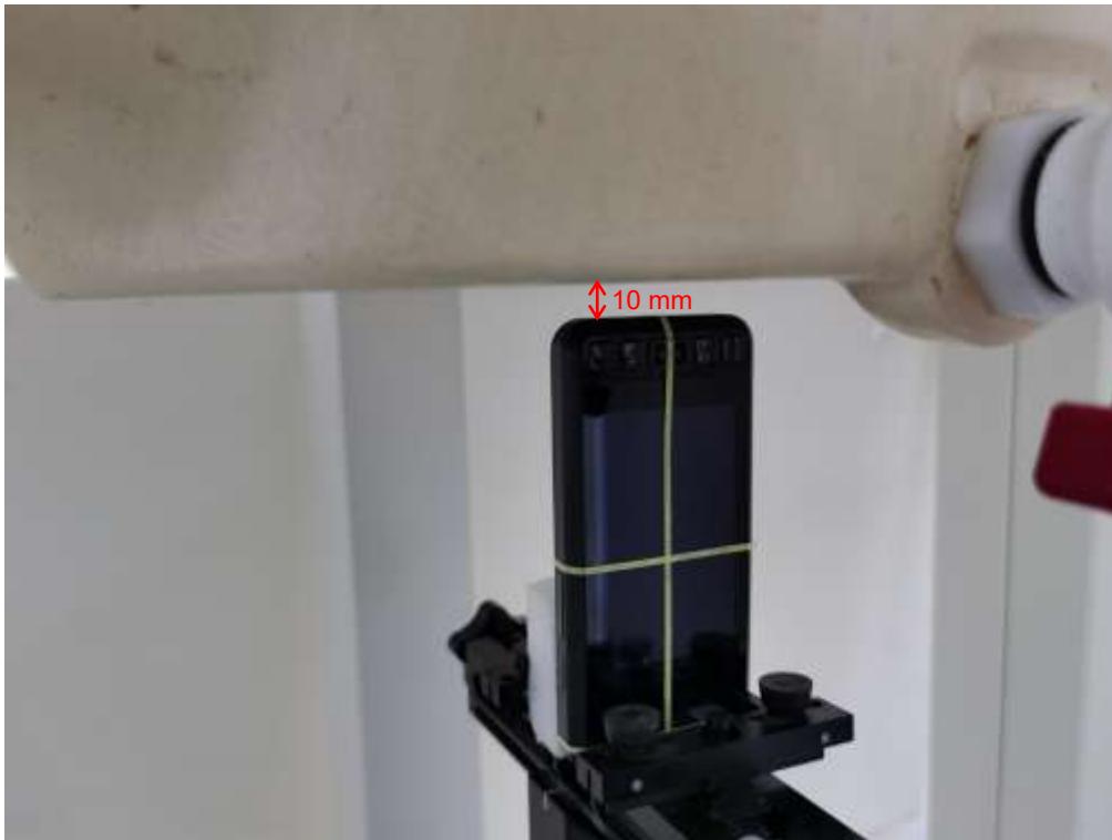
Bottom Edge (10mm)
