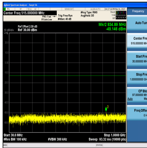
Band12-1.4MHz-QPSK-23017-6RB#0-Range1:30~1000MHz
