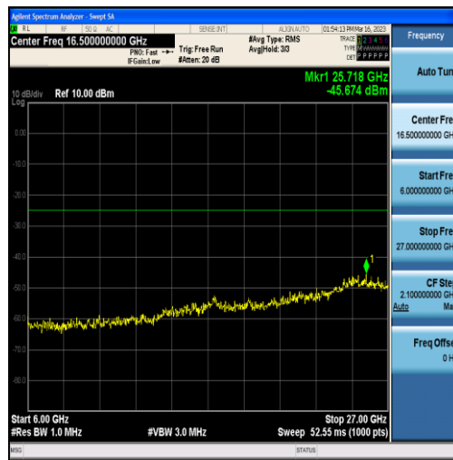
Band7-10MHz-QPSK-21100-50RB#0-Range3:6000~27000MHz
