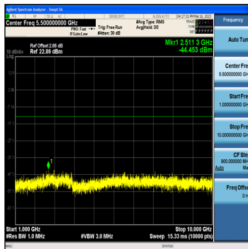
Band12-1.4MHz-QPSK-23017-6RB#0-Range2:1000~10000MHz
