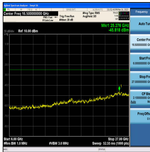
Band7-10MHz-QPSK-20800-50RB#0-Range3:6000~27000MHz
