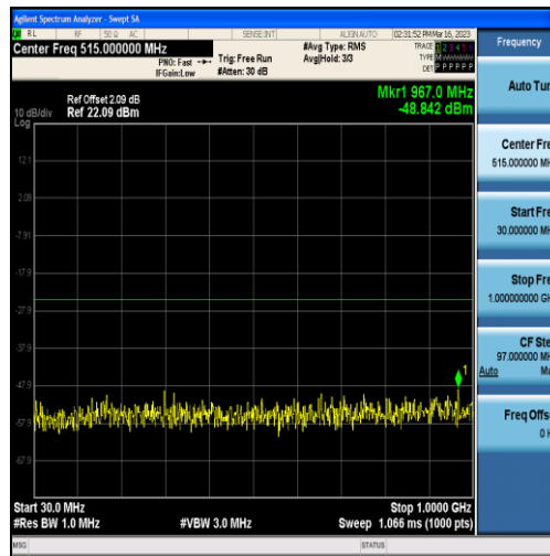
Band7-20MHz-QPSK-21350-100RB#0-Range1:30~1000MHz
