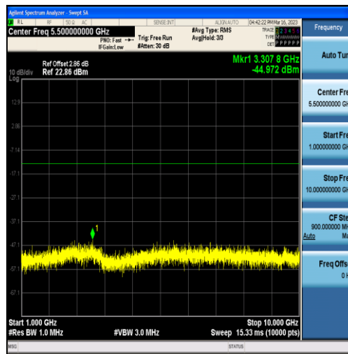
Band12-5MHz-QPSK-23095-25RB#0-Range2:1000~10000MHz
